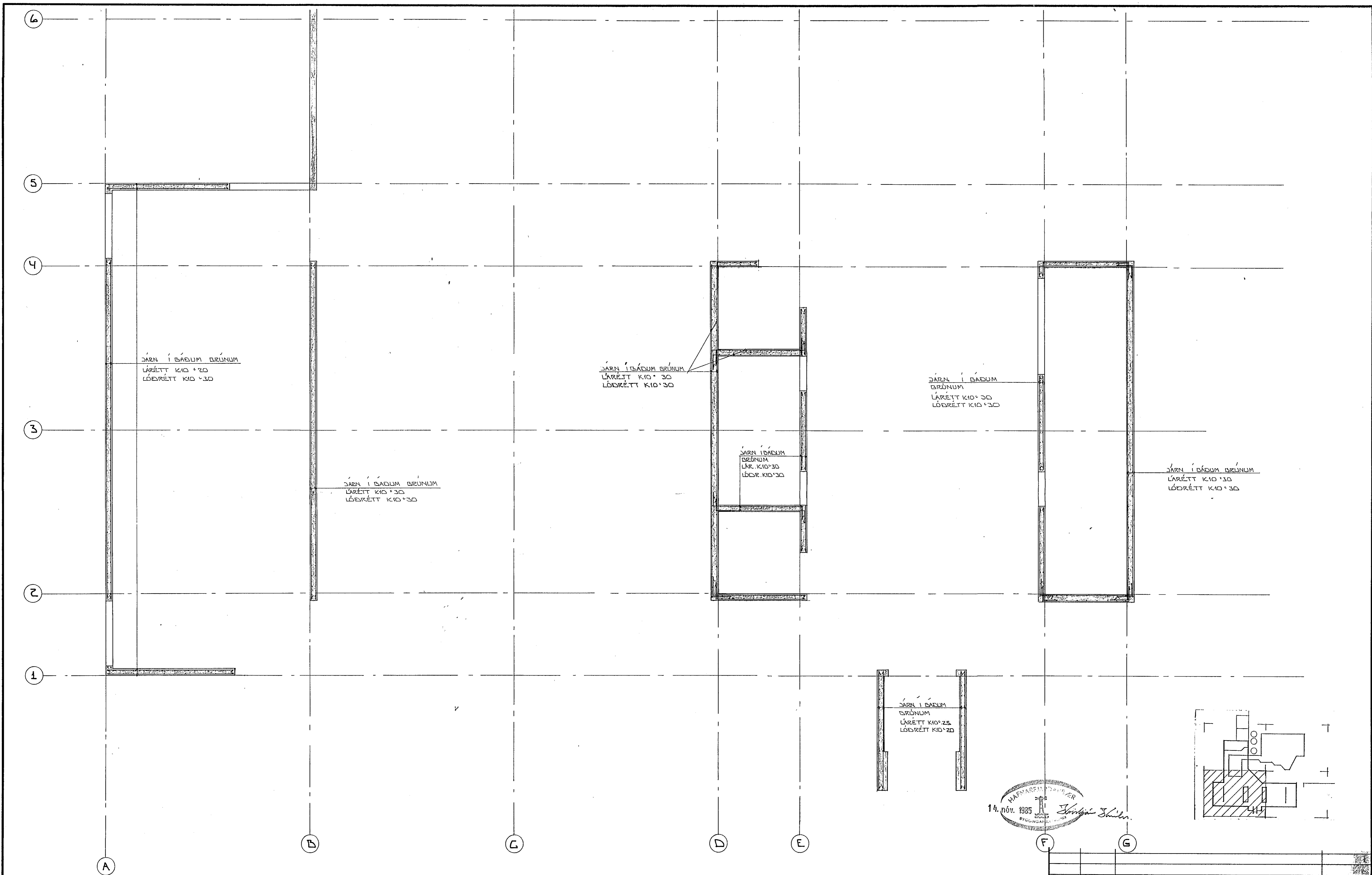
SKUNNMYND JARHVEDAR 1:50
