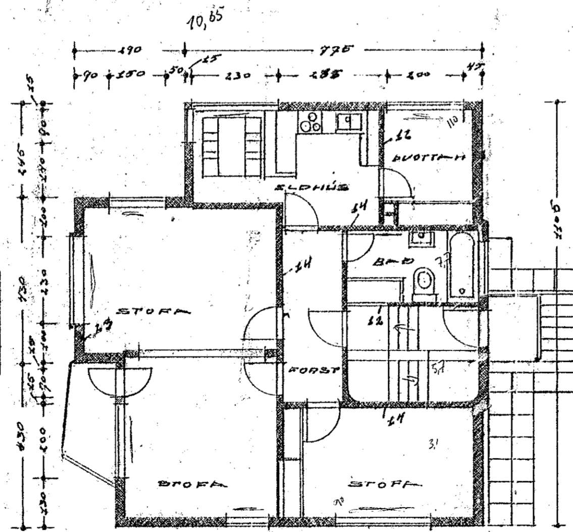
2. HÆÐ.
