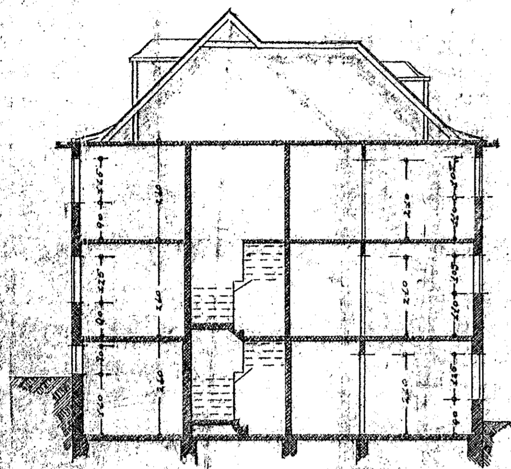
SKURÐUR
