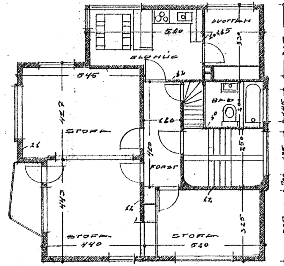
3. HÆÐ.
