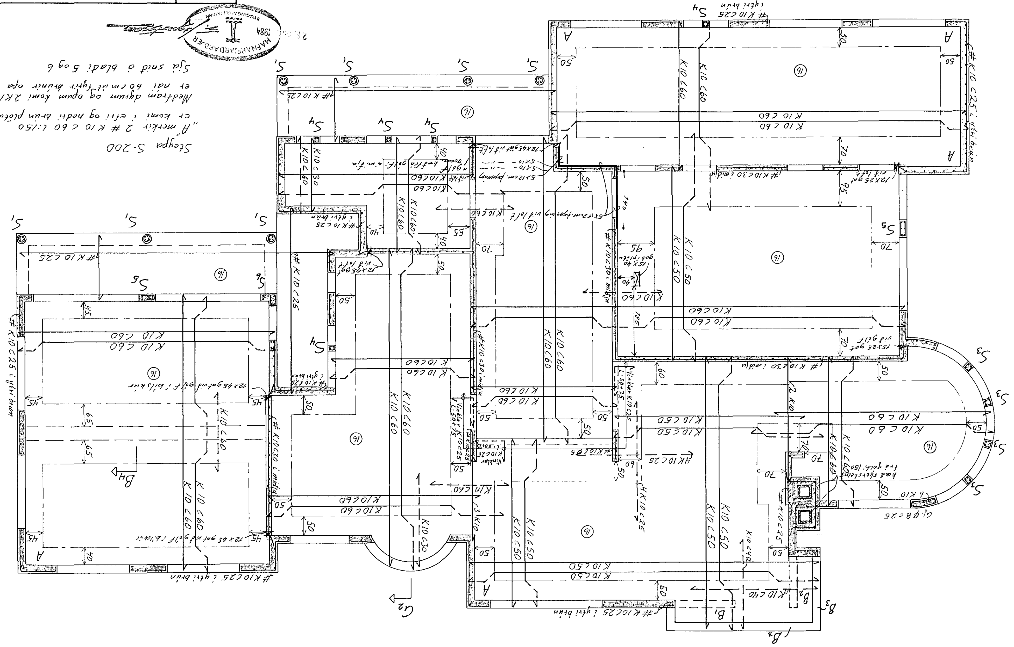
Grunnmynd hæðar 1:50
