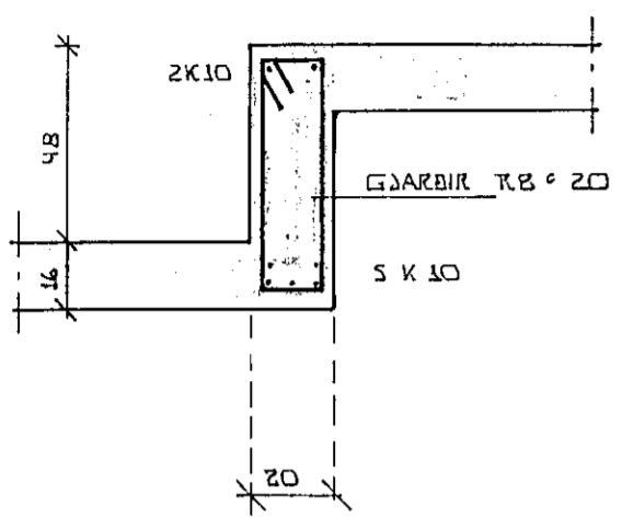
SNIÐ A 1:20
