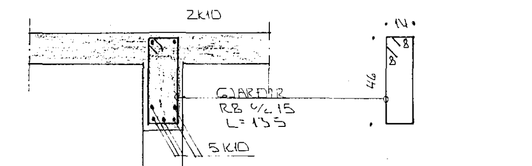
SNID YFIR BILGEYMSLUÐYRUM 1:20
