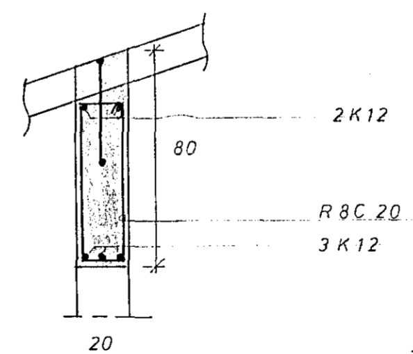
SNID I-I M 1:20
