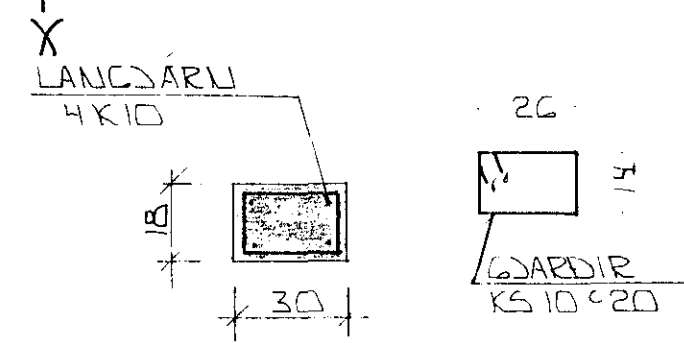
SÚLA S2 · 1:20
