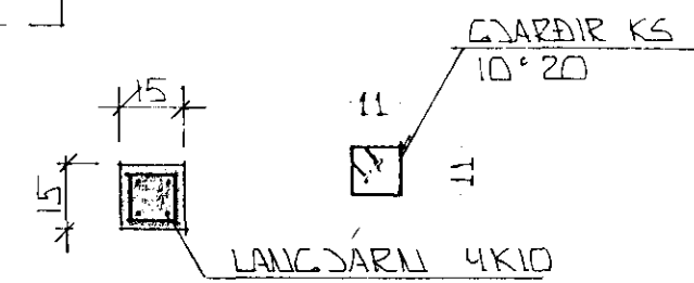
SÚLA S1 · 1:20
