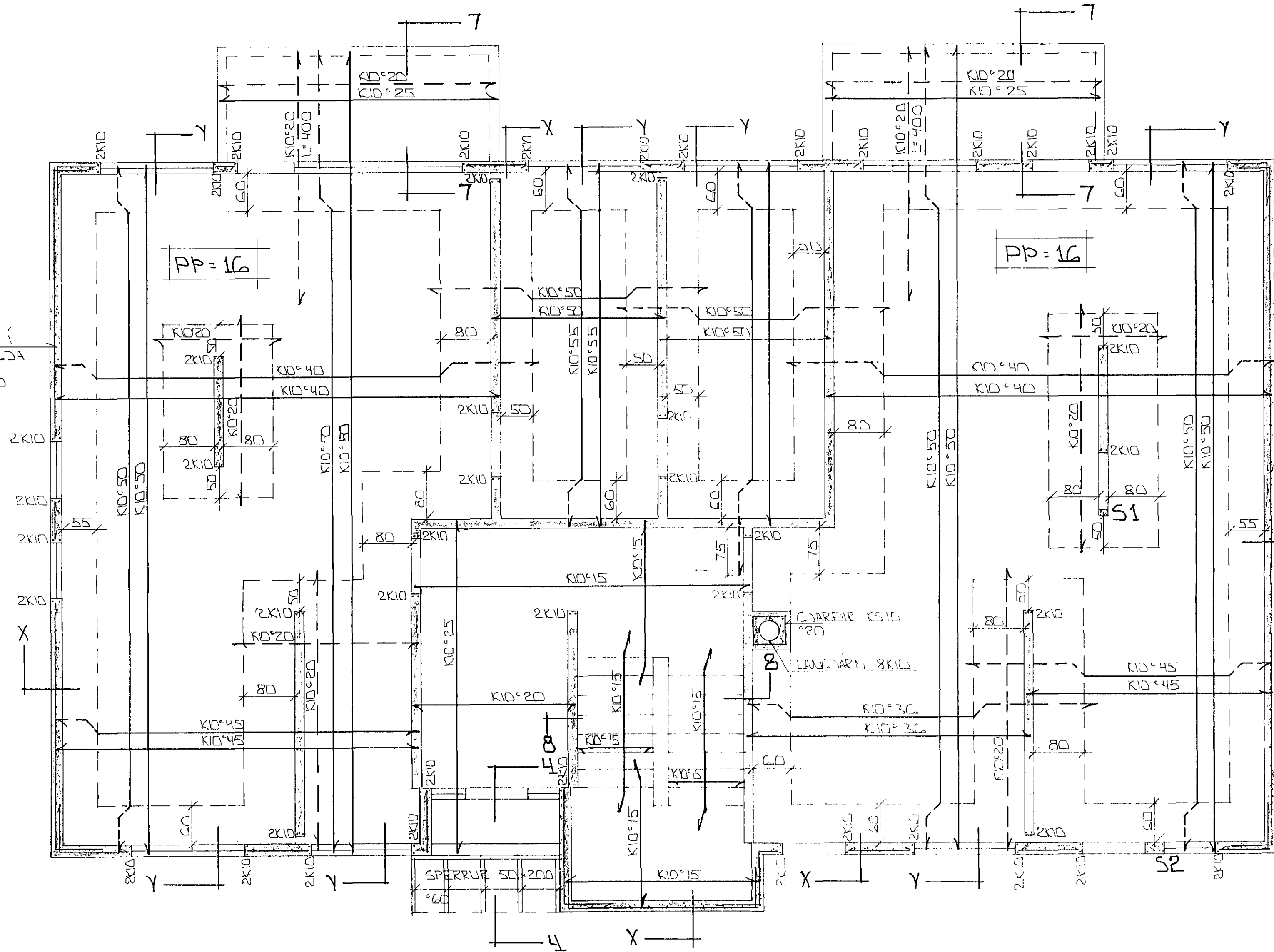
GRUNNMÝND · 1:50
