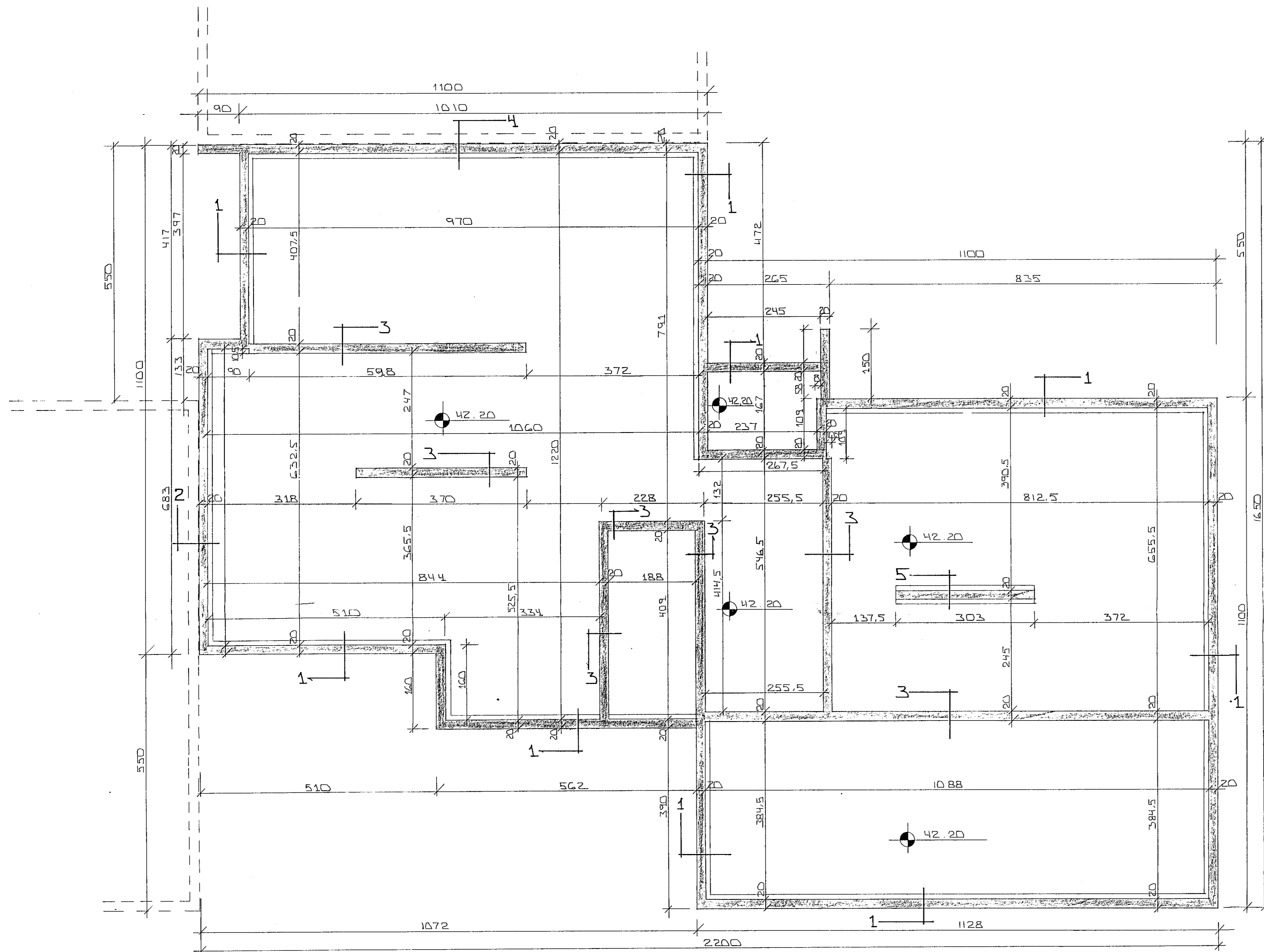
GRUNNMYND • 1 : 50
