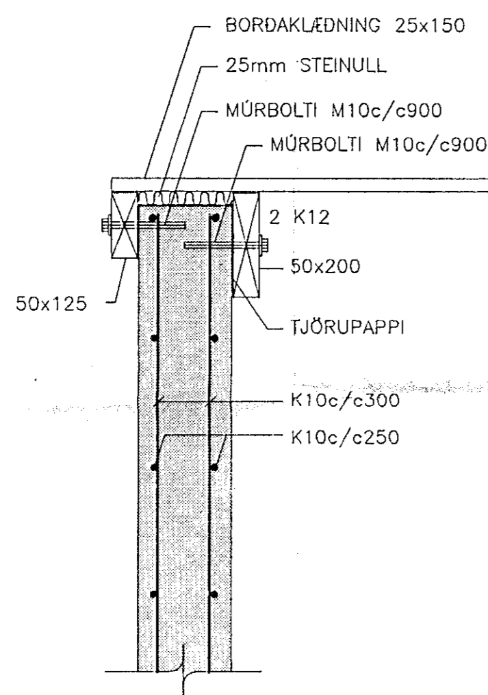
SNID G-G, 1:10
