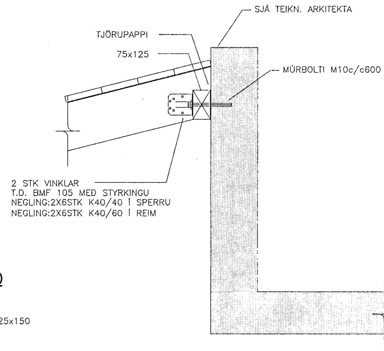
SNID G-G, 1:10
