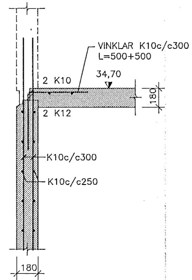
SNID A-A, 1:20
