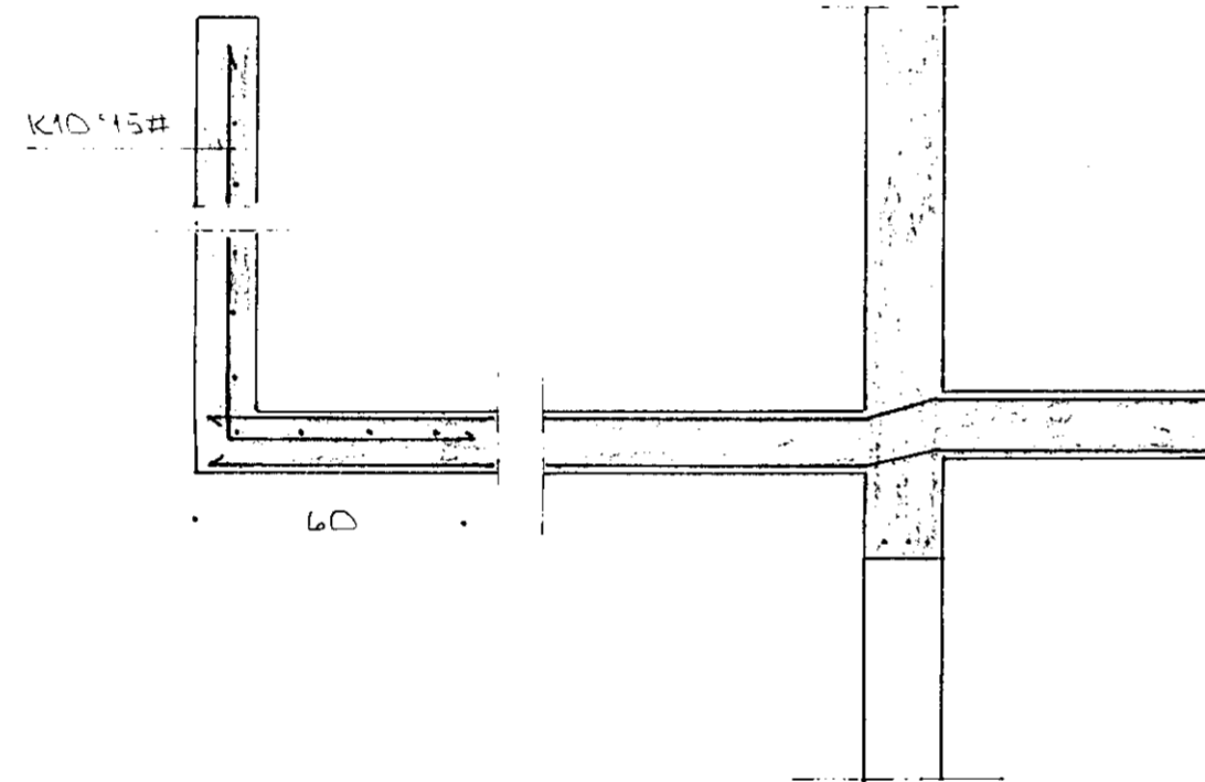
SNID 5-5 Í SVALIR ~ 1:20
