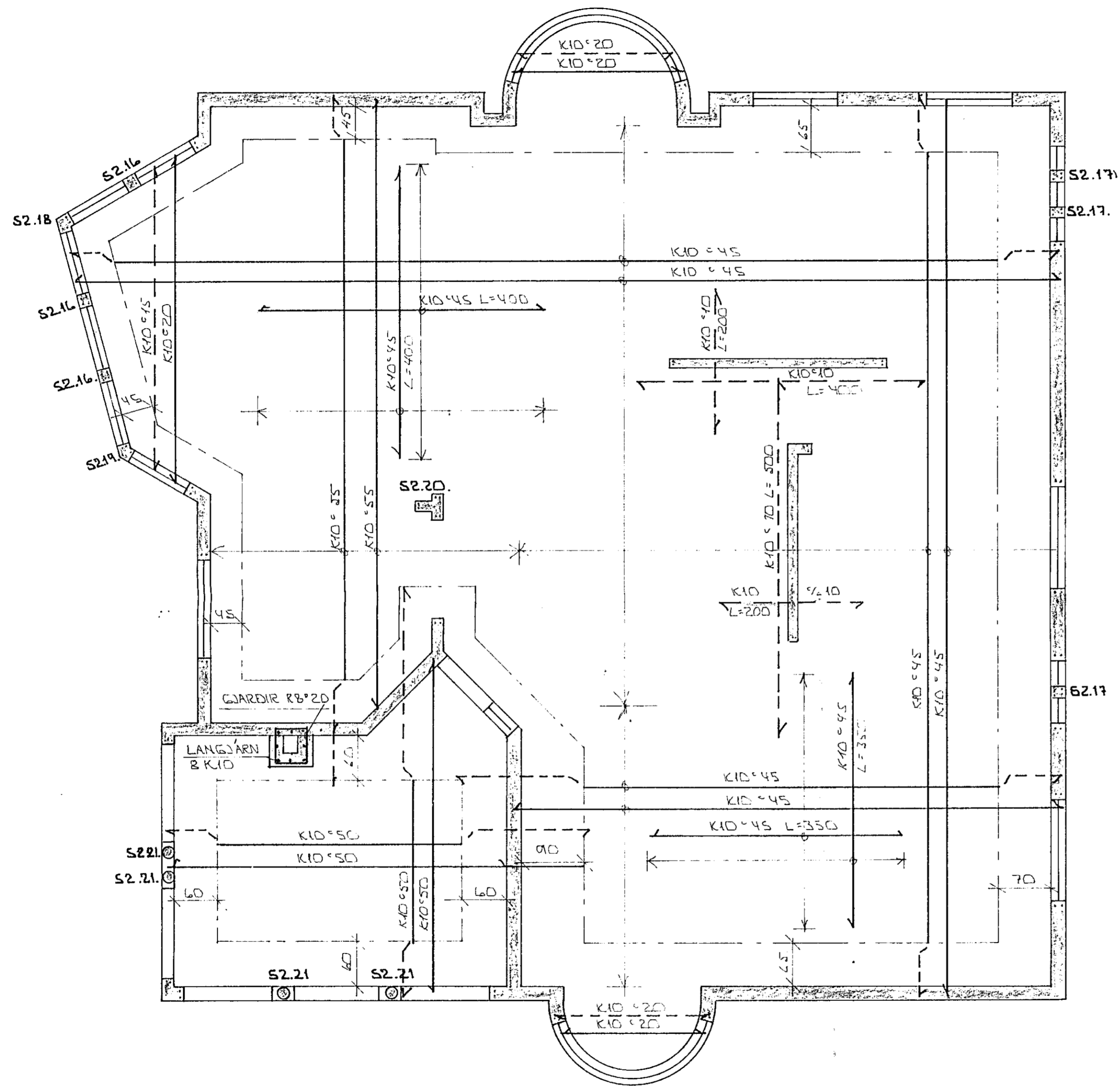
GRUNNMYND ~ 1:50
