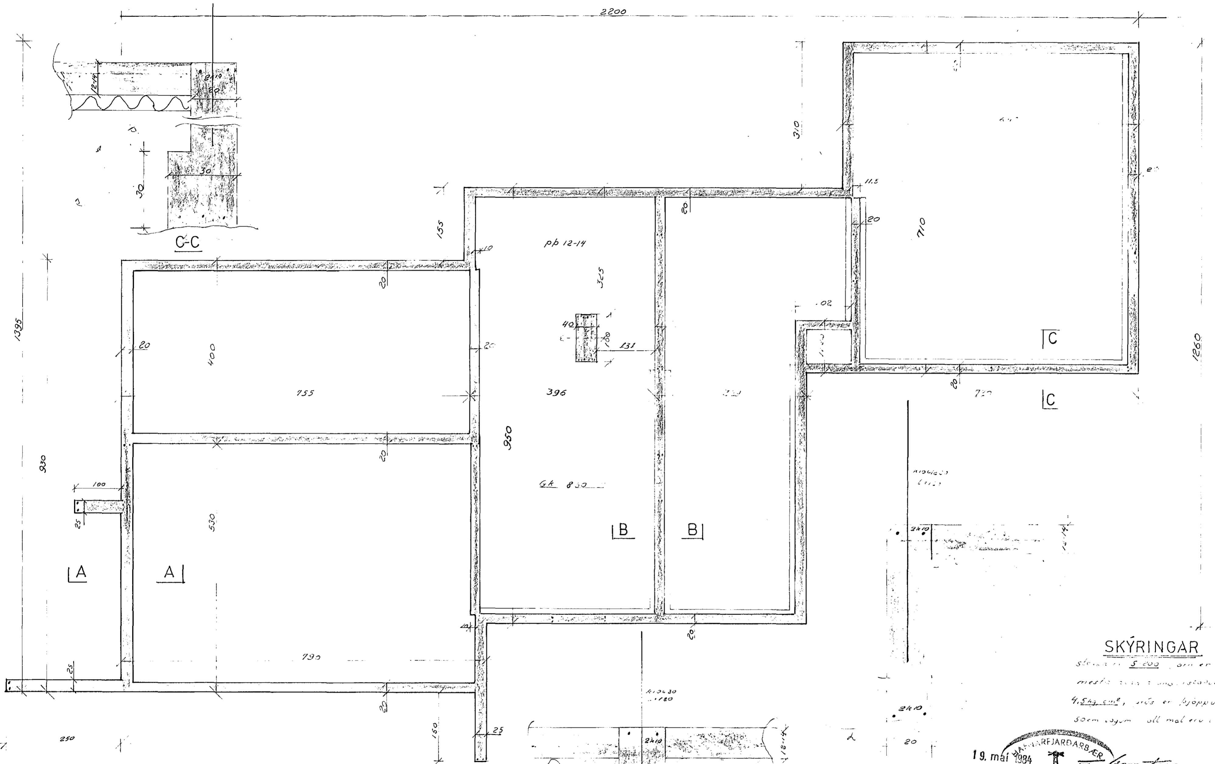
UNDIRSTÖÐUR 1:50
