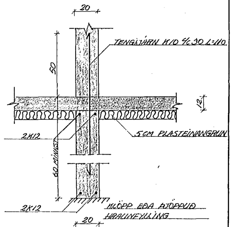
SNID D-D 1:20
