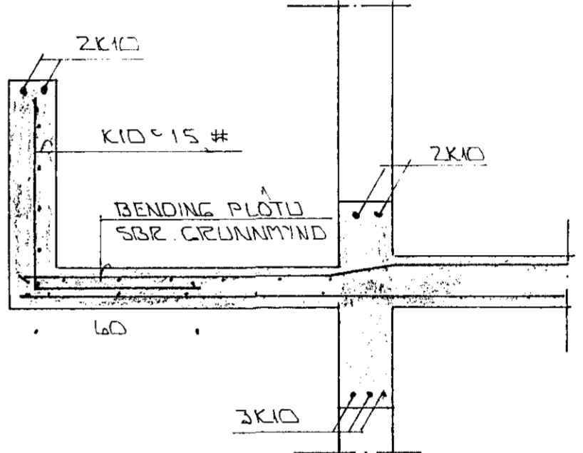
SNIED A Í SVALAR 1:20
