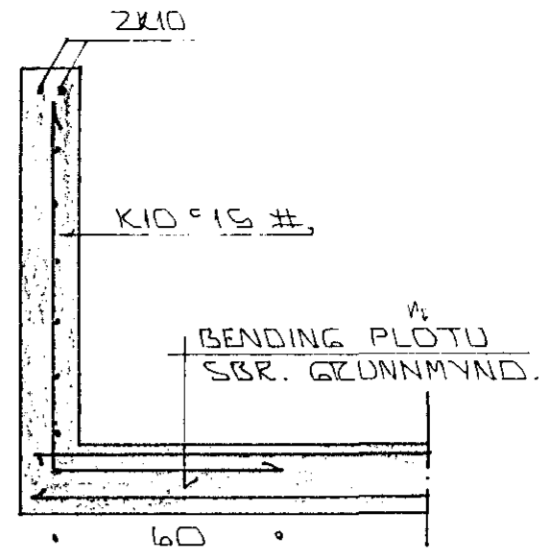
SNIED B Í HANDRÍÐ V/STIGA 1:20
