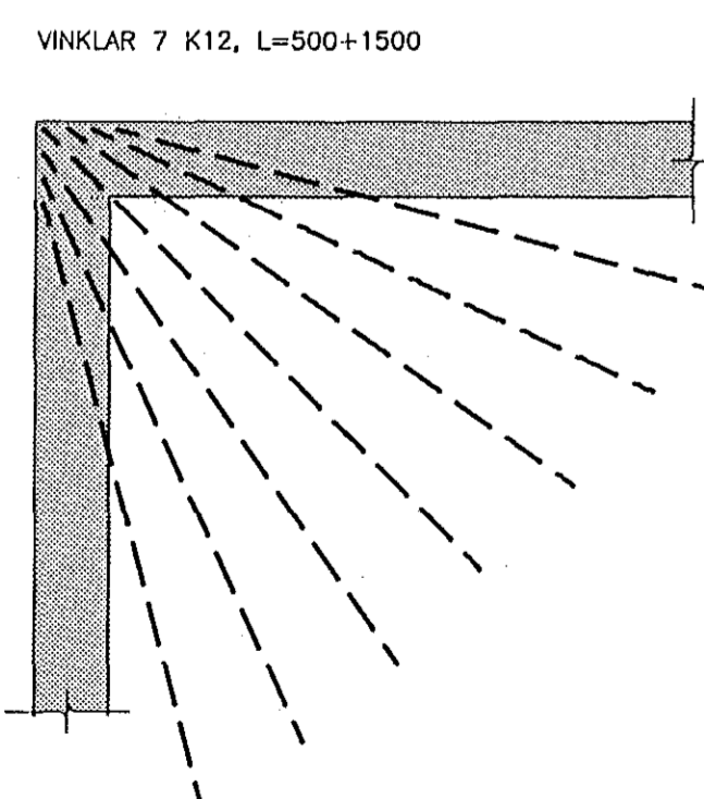
H1 HORNJÄRNUM, 1:20
