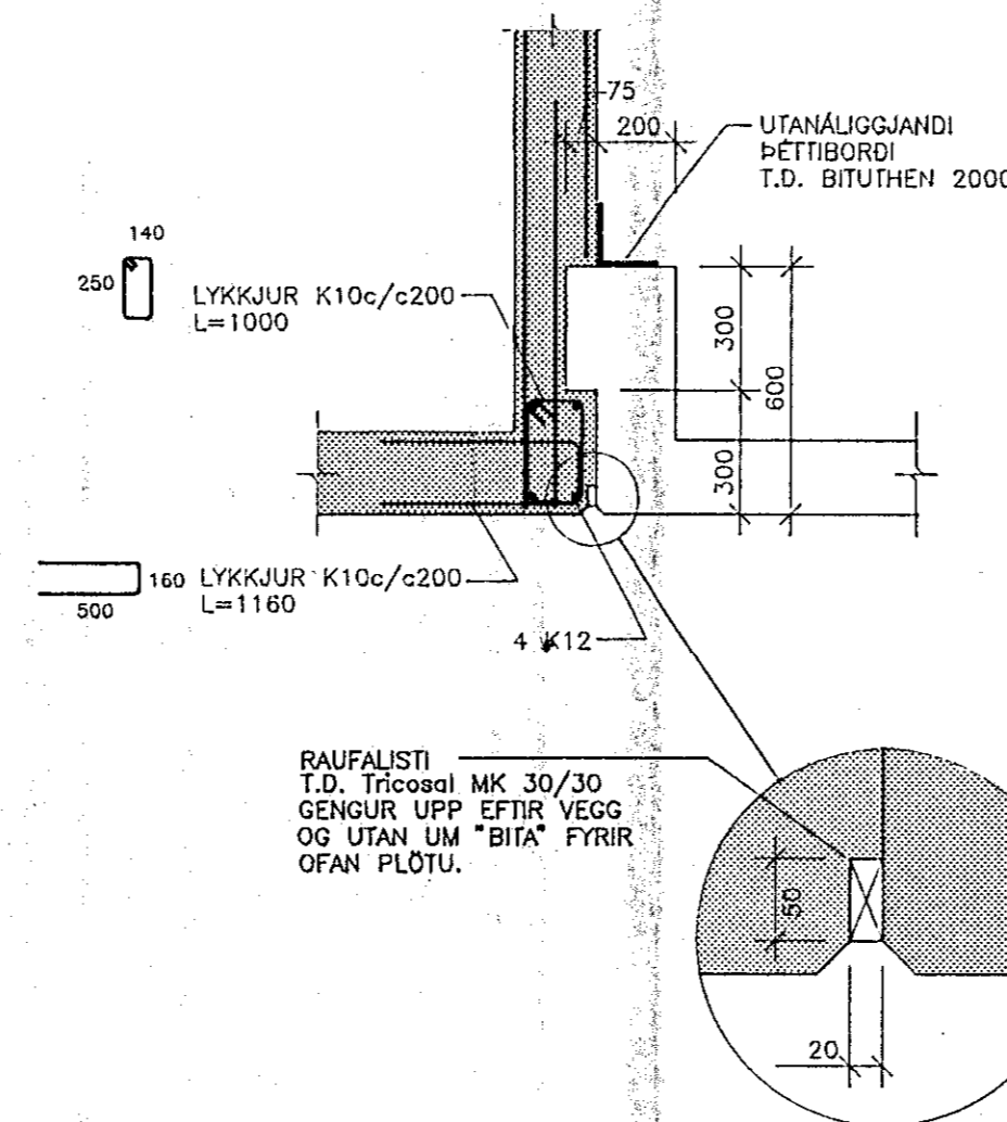
DEILI D-3. 1:20
