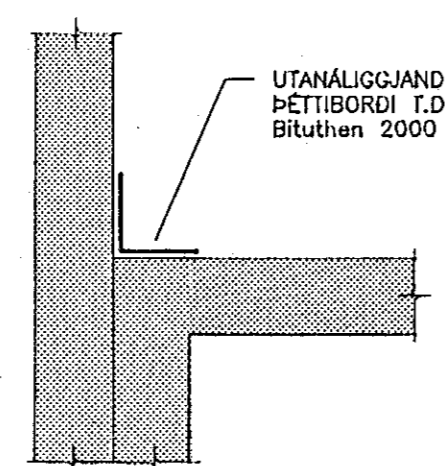
DEILI D-2. 1:20
