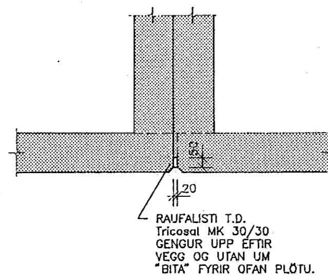
DEILI D-1. 1:20
