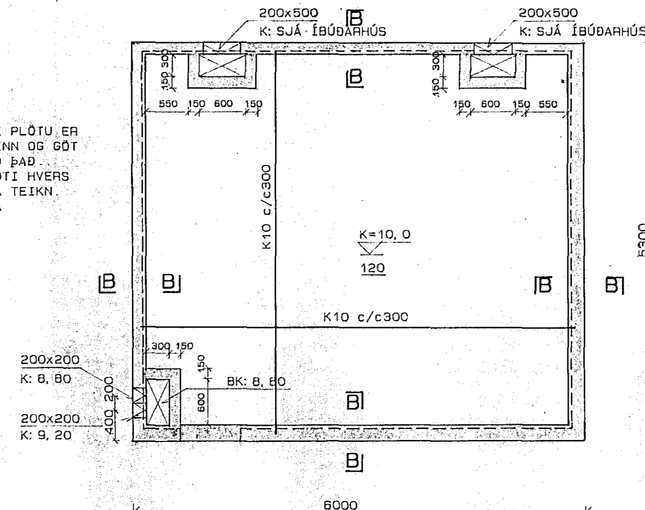
GRUNNMYND, 1: 50
