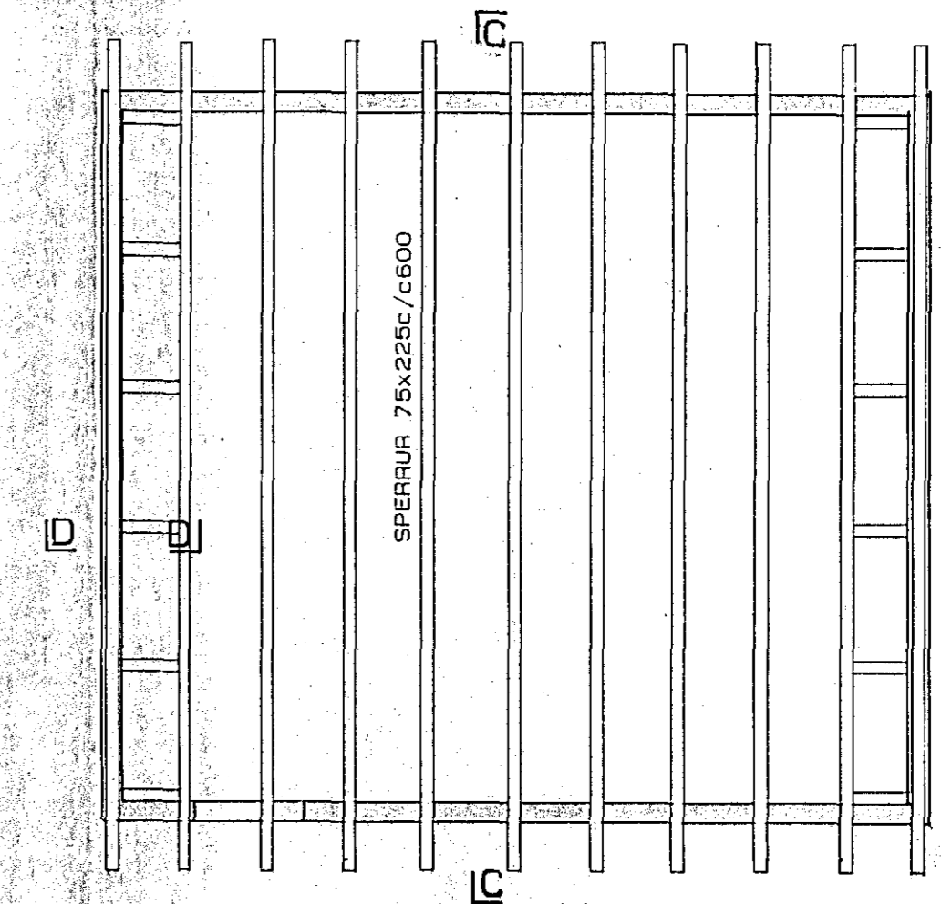
ÞAK: GRUNNMYND, 1: 50
