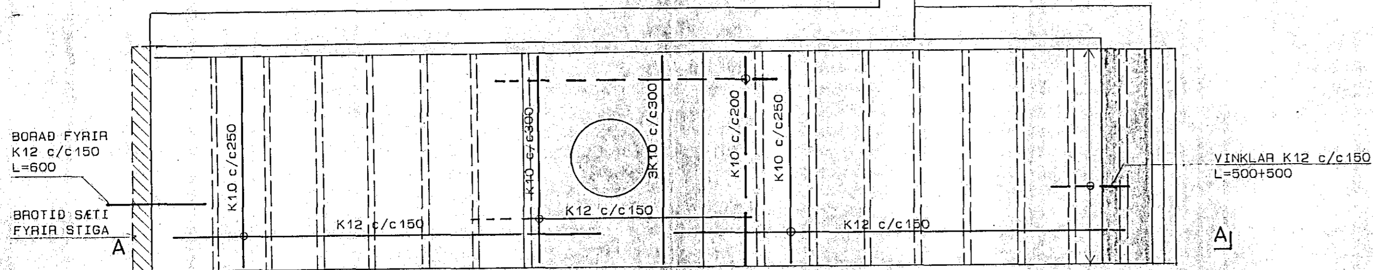
GRUNNMYND, 1: 20
