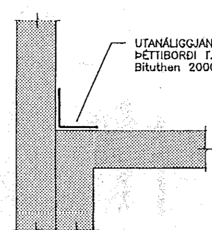
DEILI D-2. 1:20
