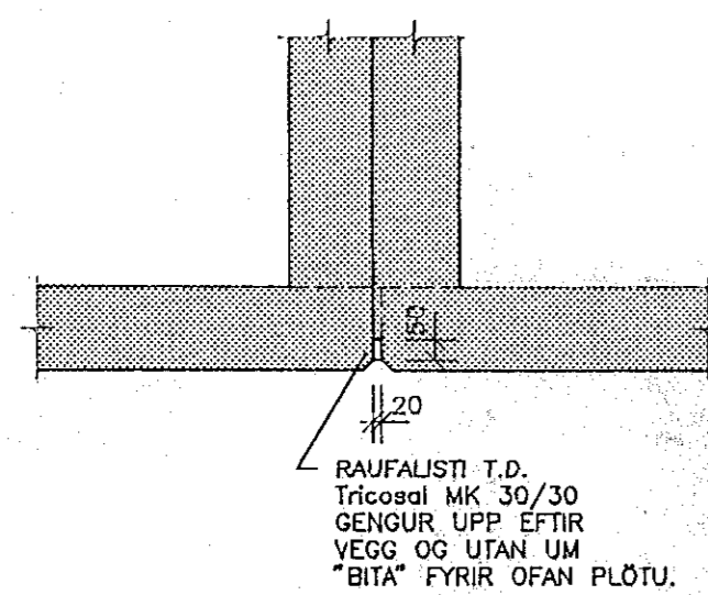
DEILI D-1. 1:20
