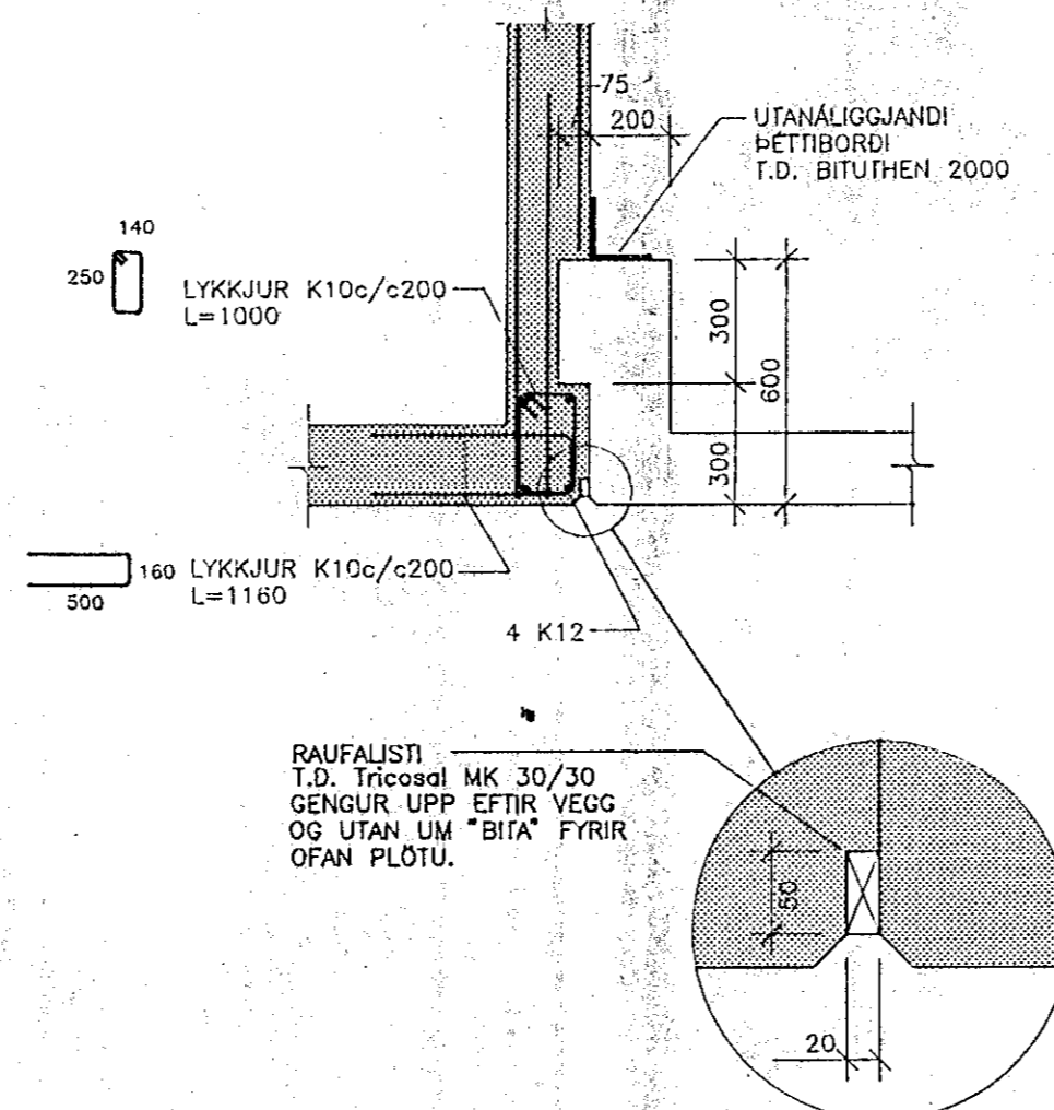
DEILI D-3. 1:20
