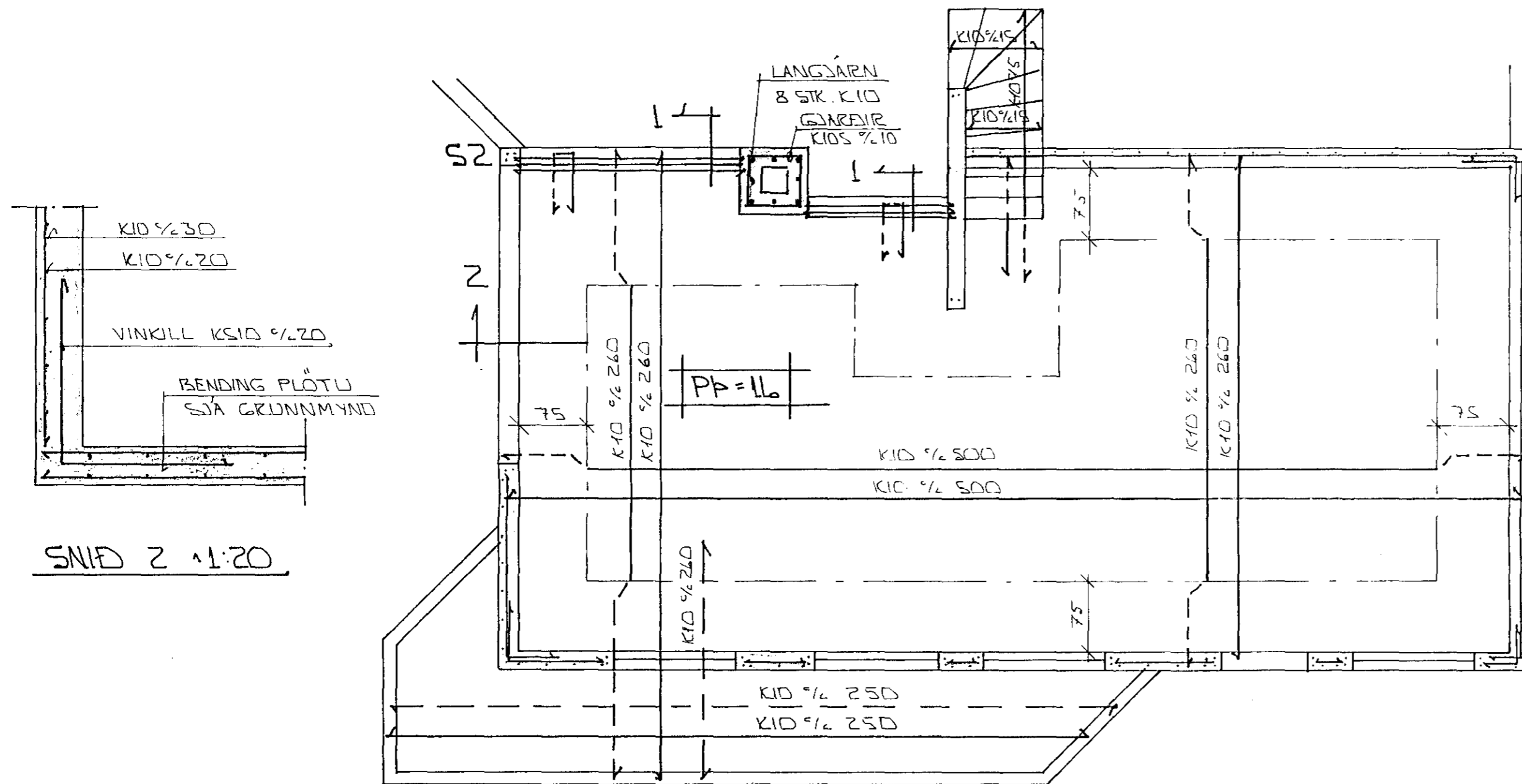
GRUNNMYND 1:50
