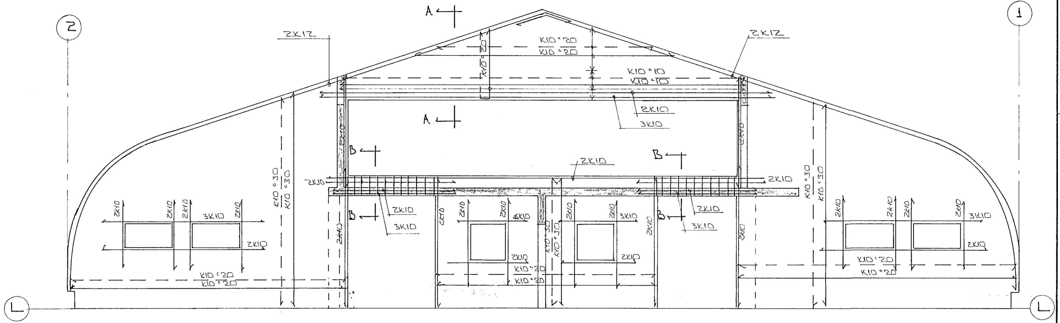
ÁSYND Á ÚTVEGG (MODULLÍNA L) 1:50
