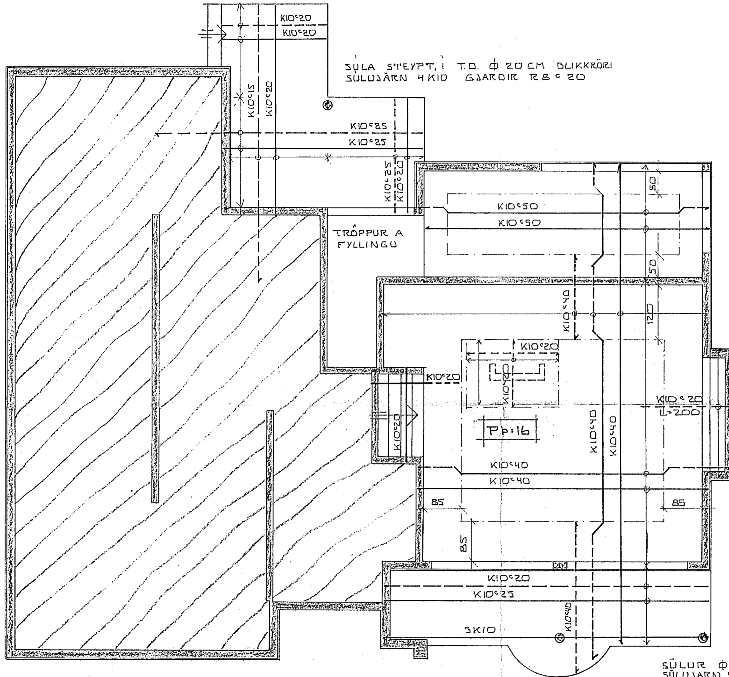
GRUNNMYND - KJALLARA 1:50
