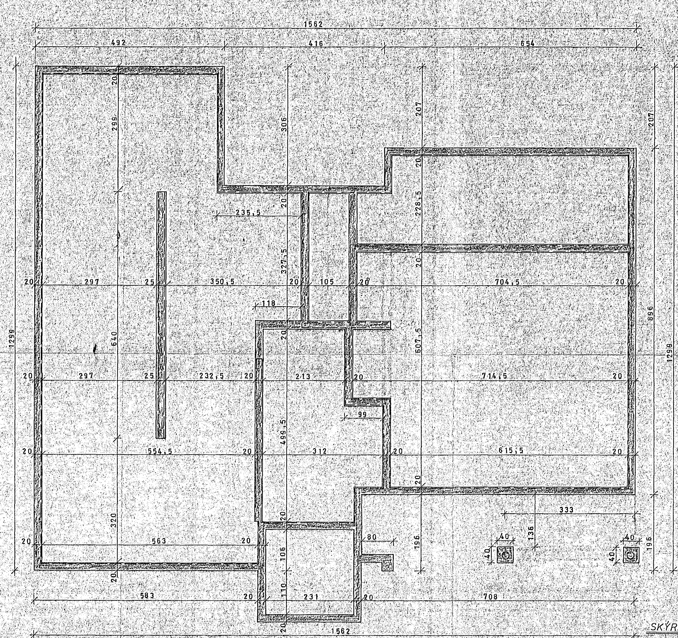
GRUNNMYND - UNDIRSTÖÐUR 1:50
