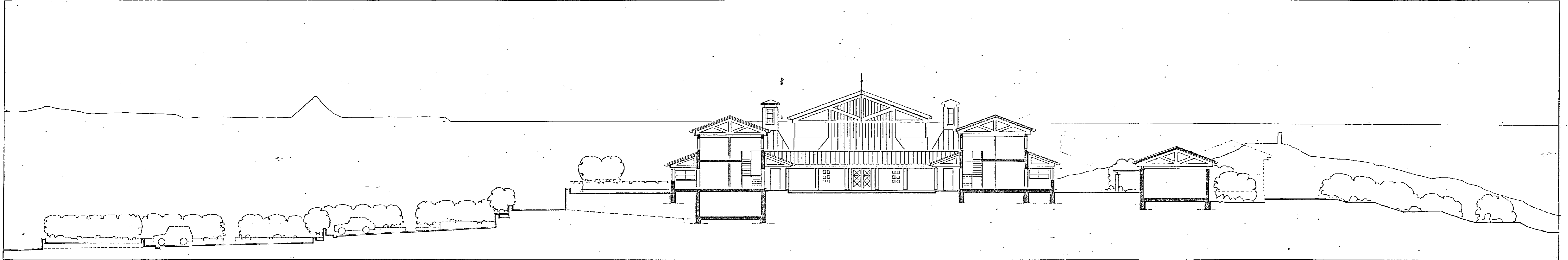
SKURÐUR AA
