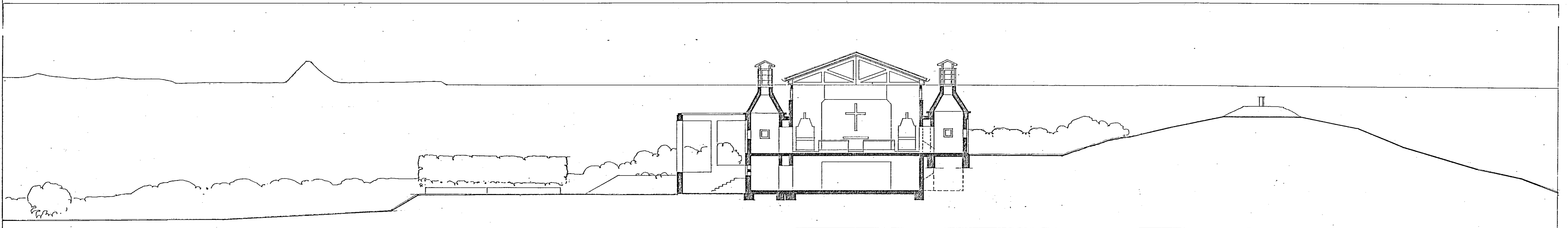
SKURÐUR BB
