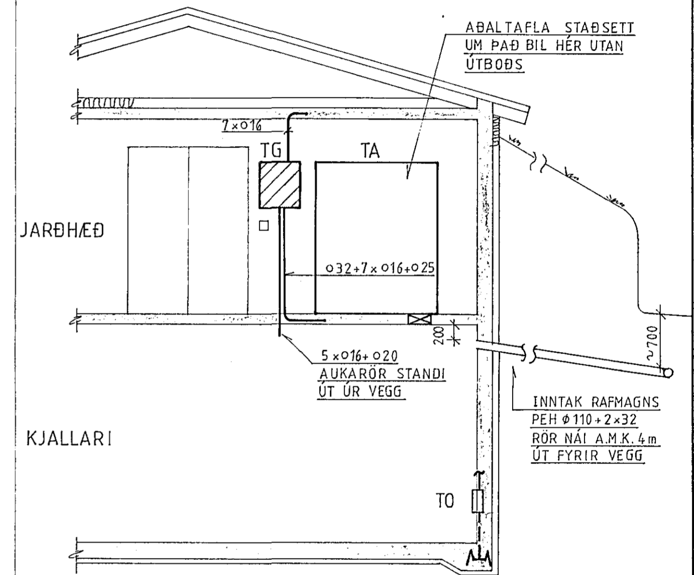
SNIÐ A-A, 1:50
