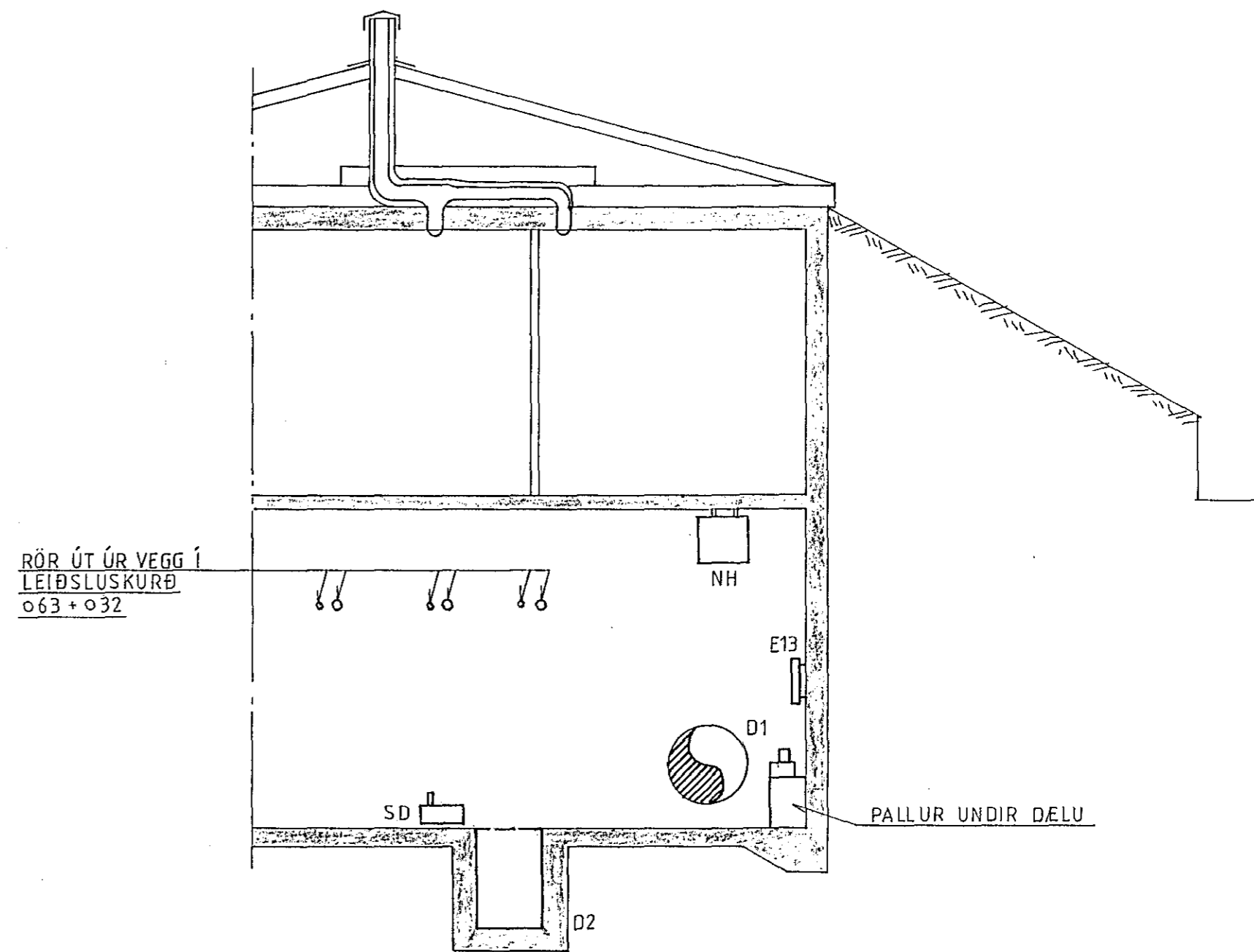
SNIÐ A-A, 1:50
