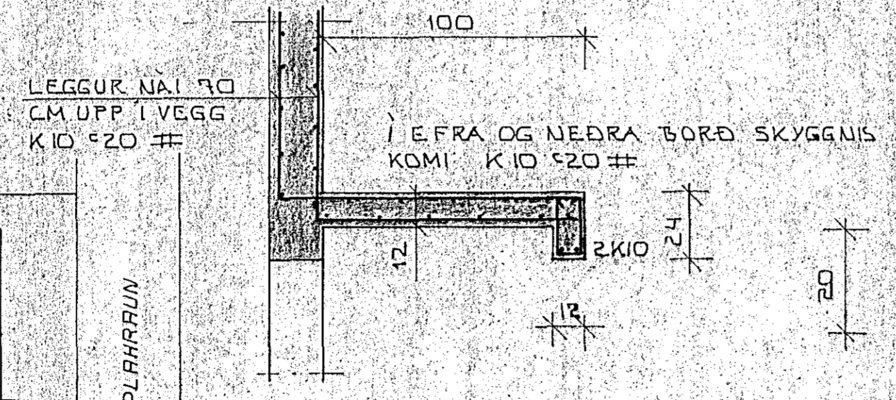
SNID A-A 1:20
