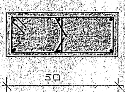
SÚLA S.1 15STK 1:10
