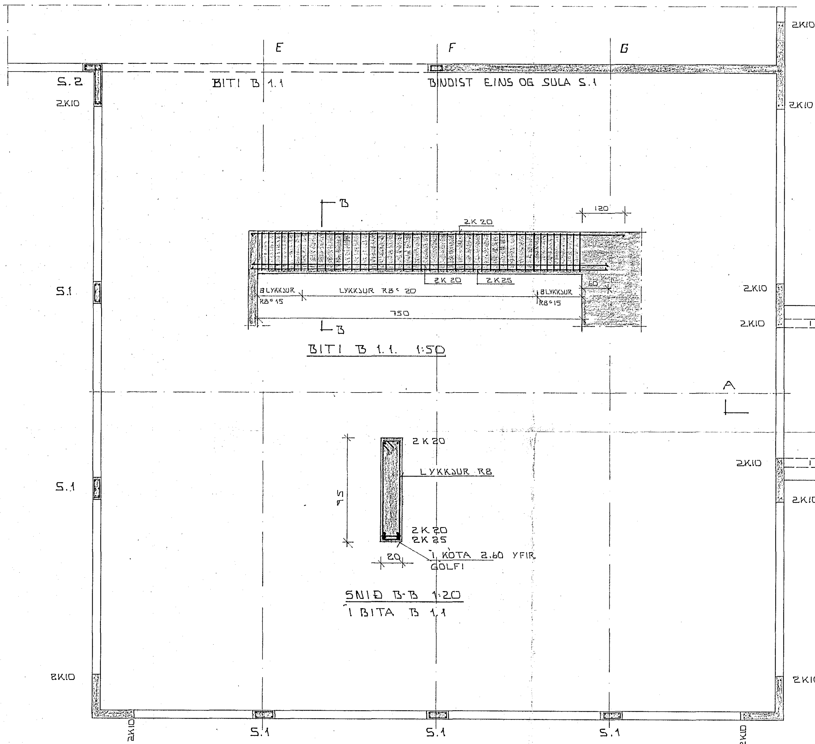
GRUNNMYND 1:50
