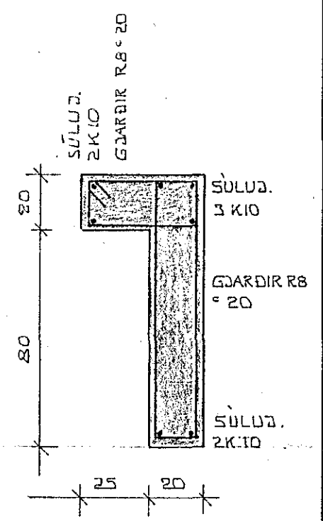
SÜLA S.2 1:20
