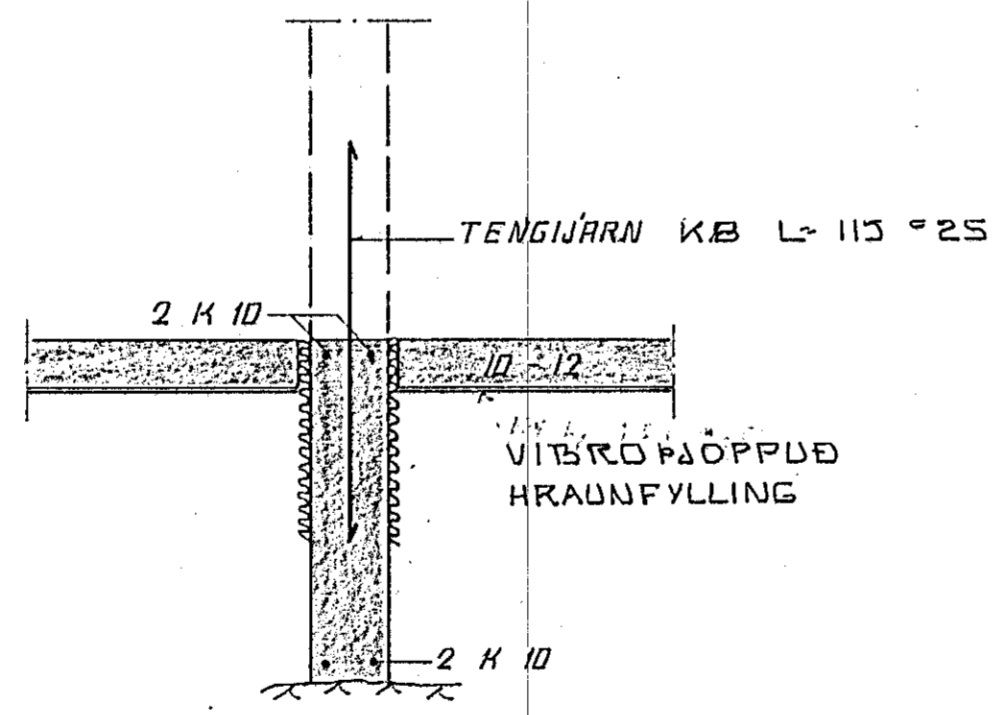
SNID 1 INNVEGG 1:20
