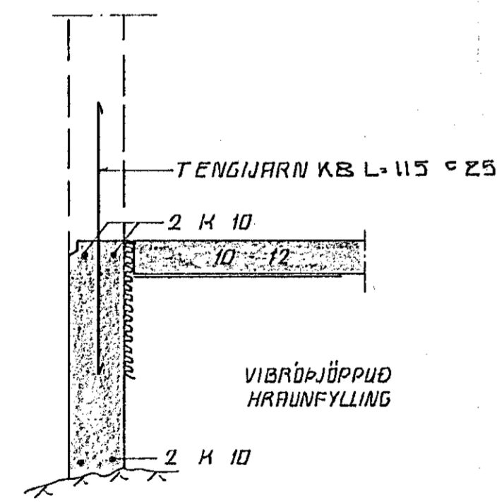
SNID 1 ÚTVEGG 1:20
