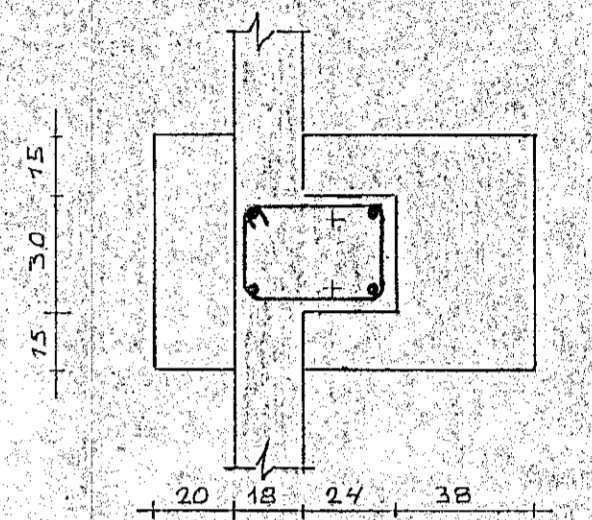
SNID D-D 1:20
