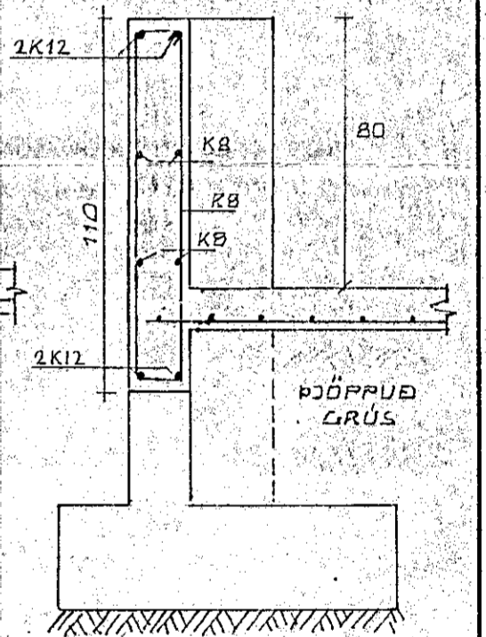
SNID D-D 1:20
