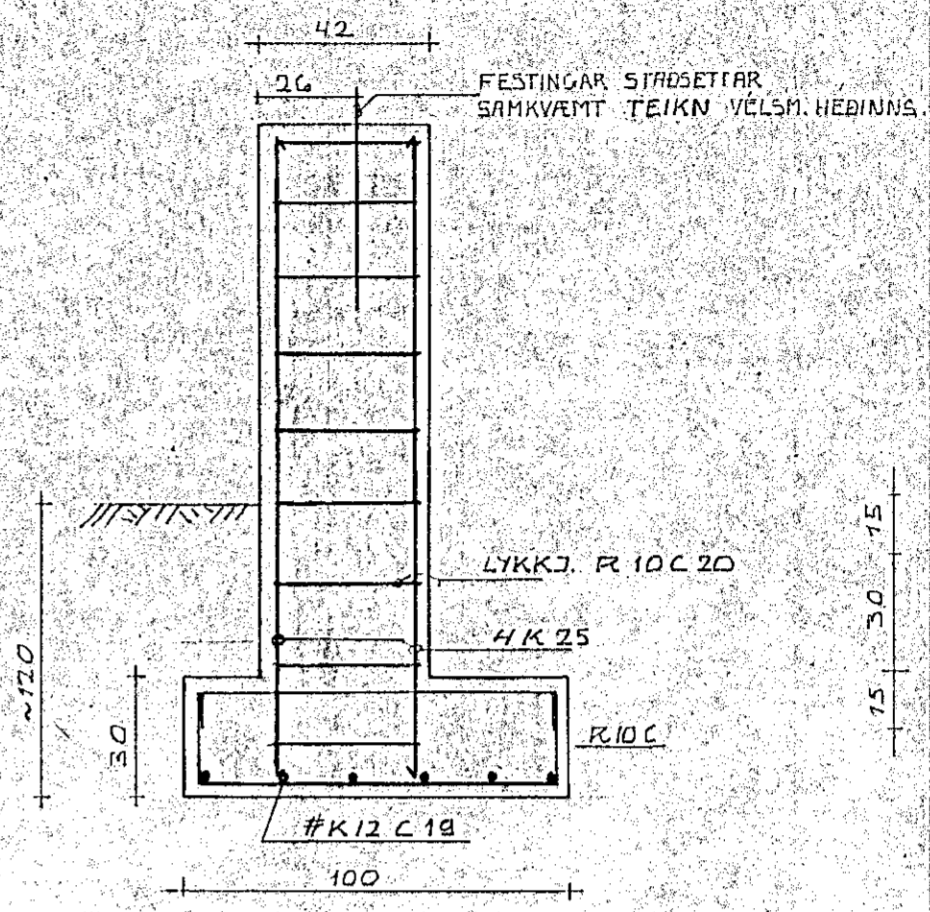
SNID A-A 1:20
