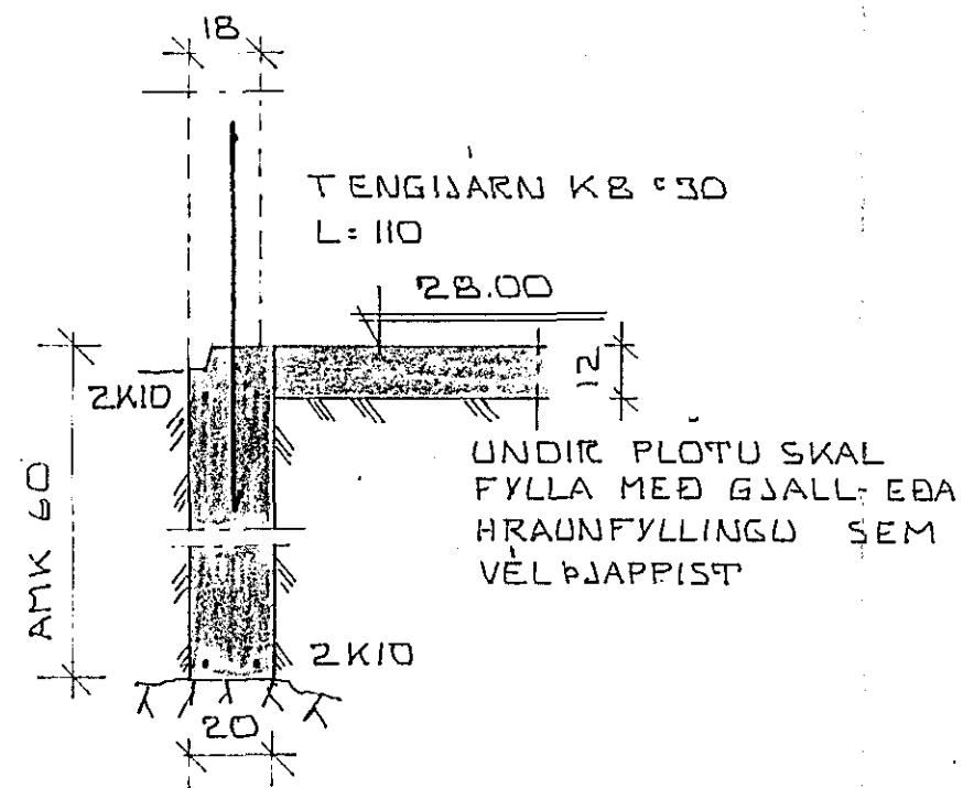
SNID Í UNDIRSTÖÐUR 1:20
