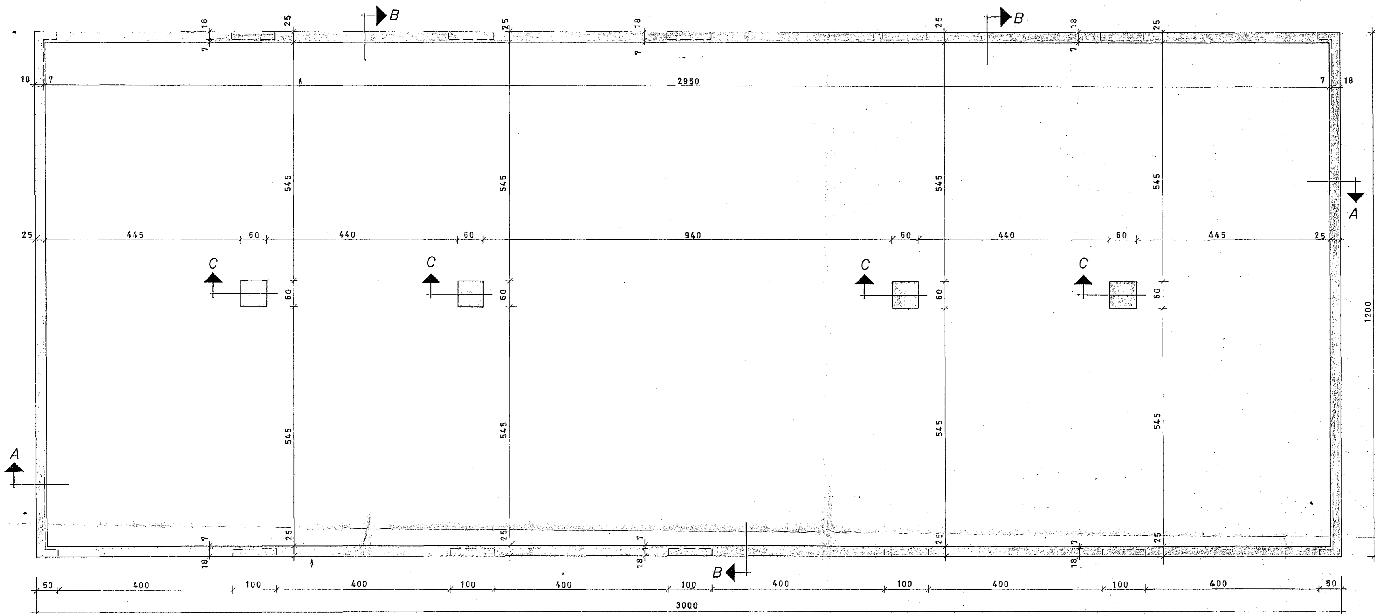
GRUNNMYND - UNDIRSTÖÐUR 1:50
