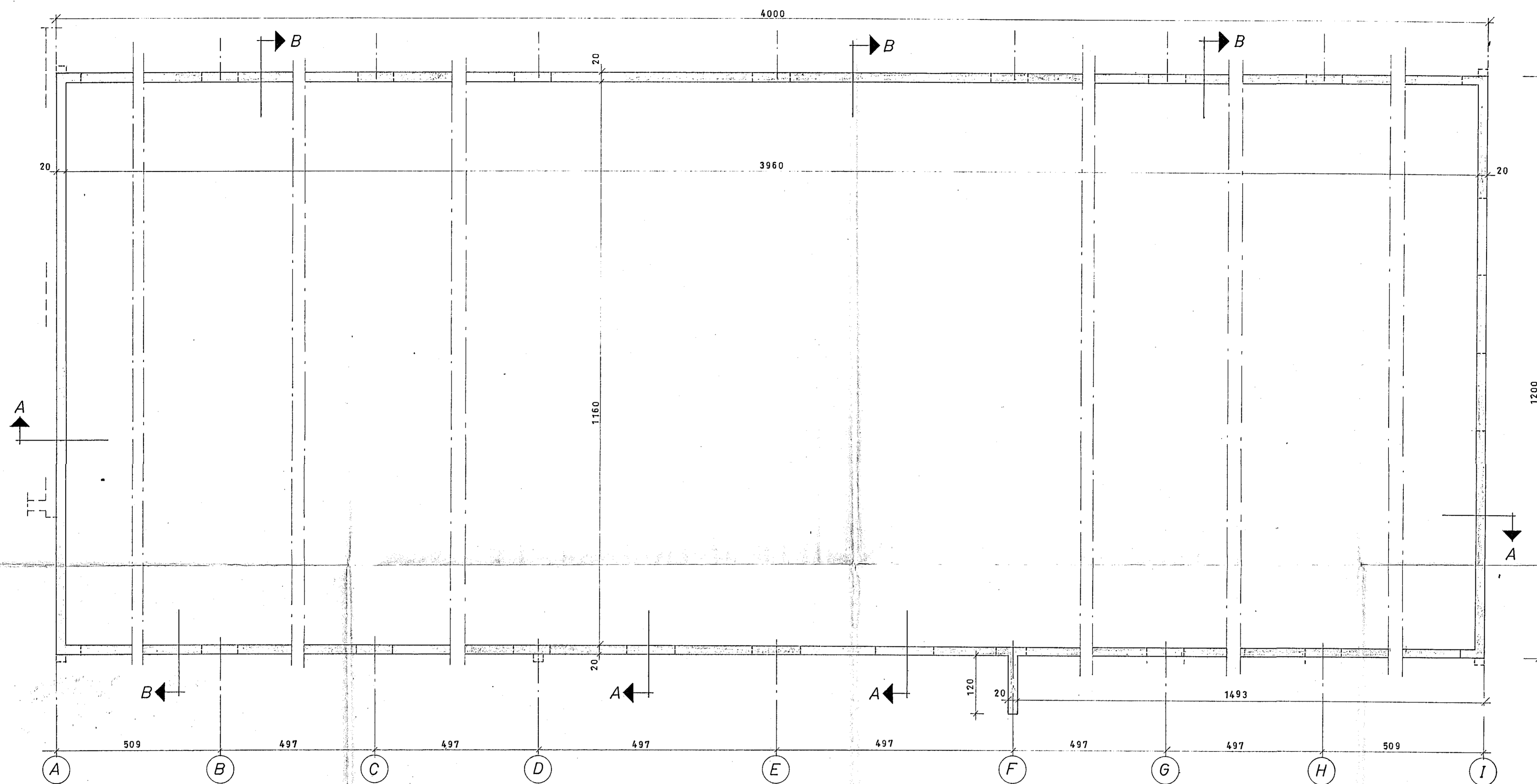
GRUNNMYND – UNDIRSTÖÐUR 1:50
