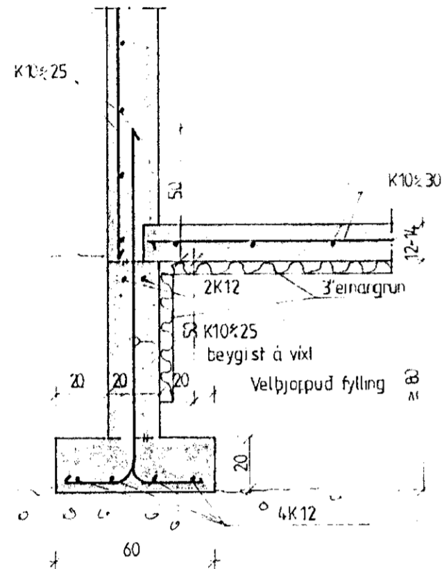
Snid A1 - A1 1:20
