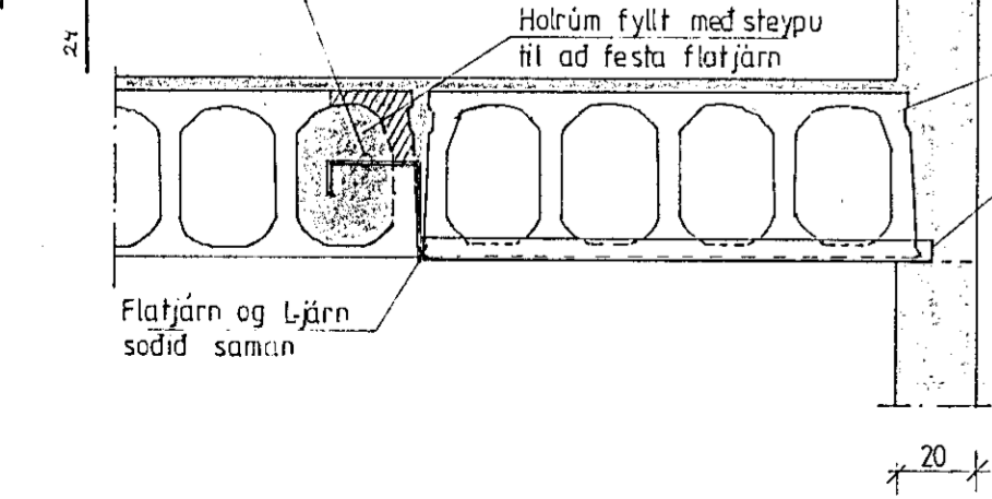
Snið A1- A1 1:20
