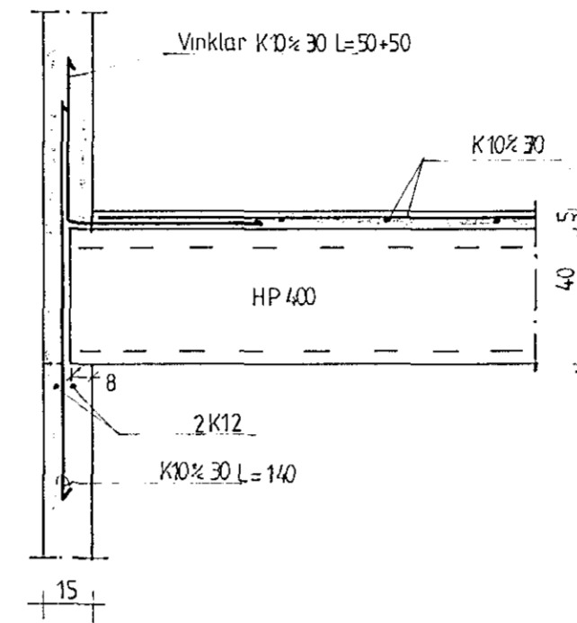
Snid C3 - C3 1:20
