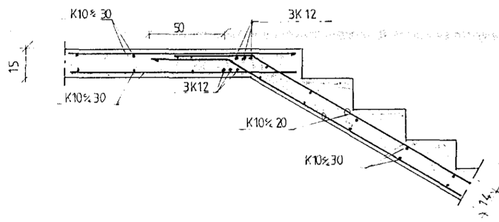
Snid C4 - C4 1:20
