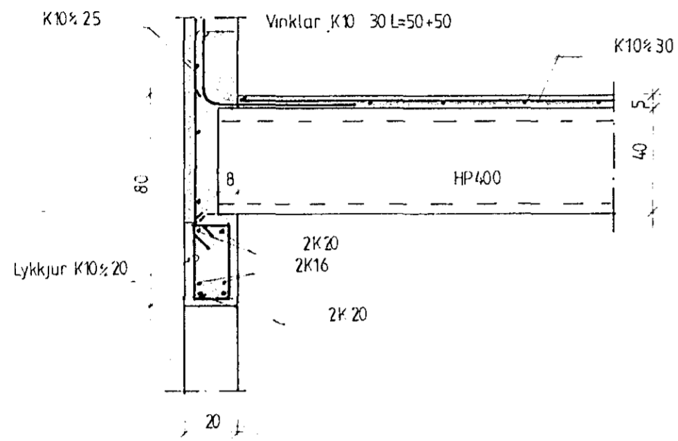
Snid C1 - C1 1:20
