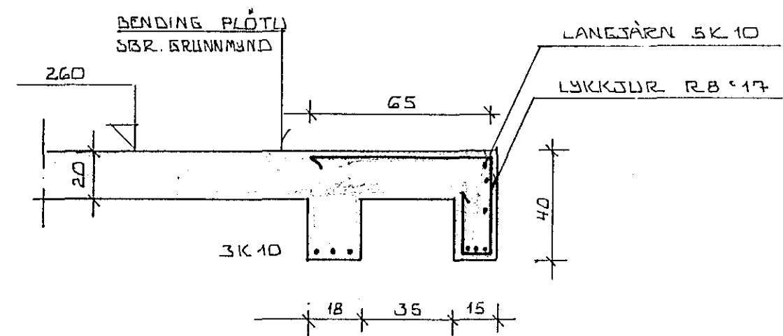
SNID A-A ~ 1:20
