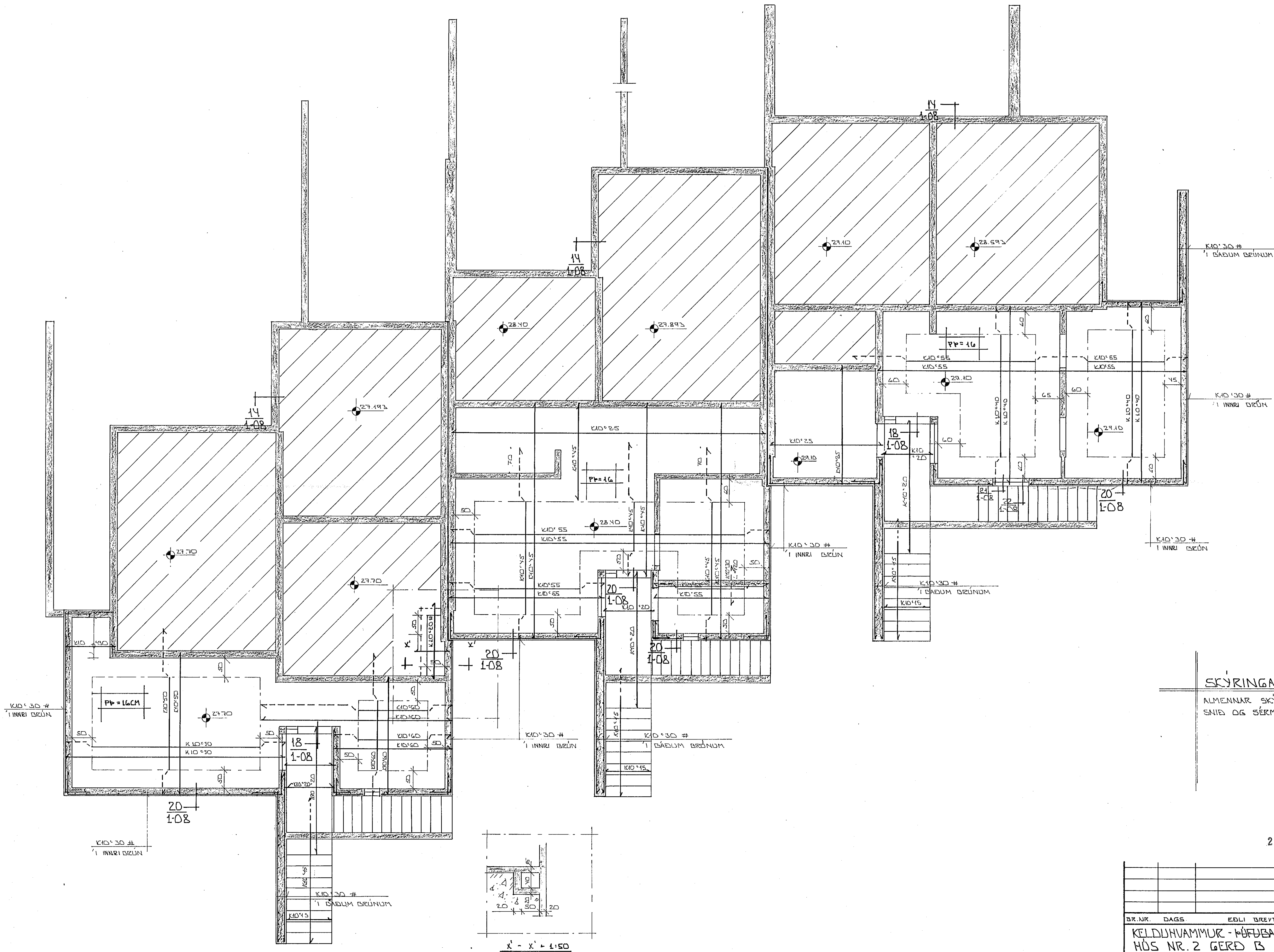
GRUNNMÝND ~ 1:50
