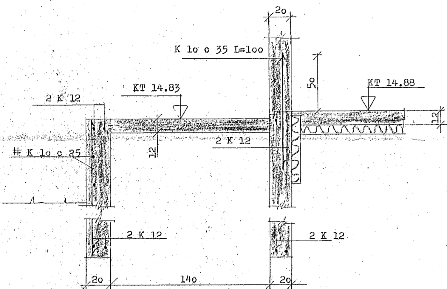
SNID G-G 1:20
