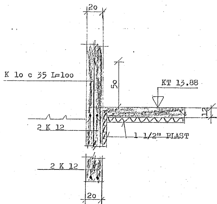
SNID G-G 1:20
