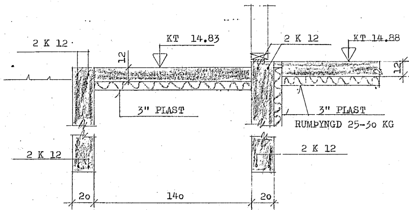
SNID D-D 1:20
