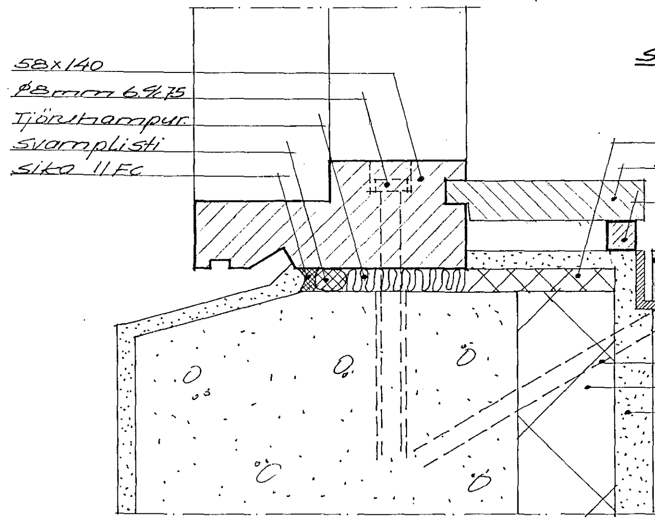
Snið A6-A6 M1:2
