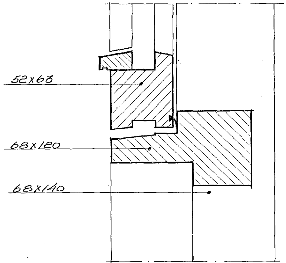
Snið A3-A3 M1:2
