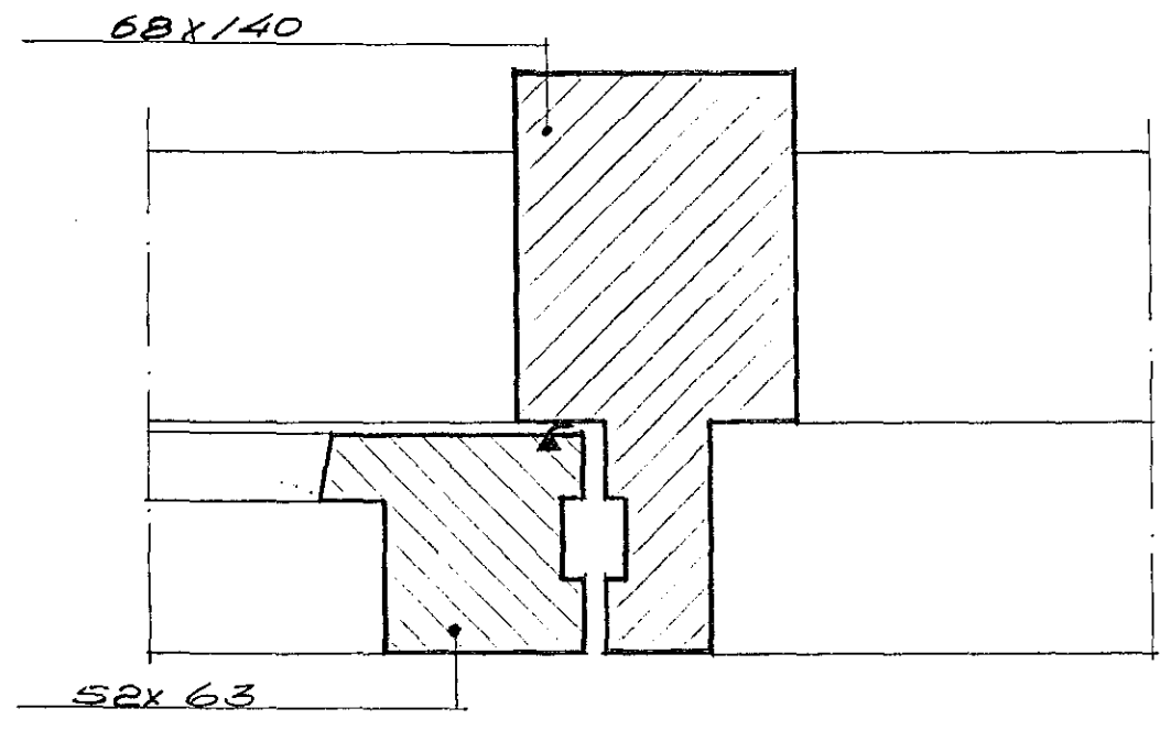
Snið A4-A4 M1:2
