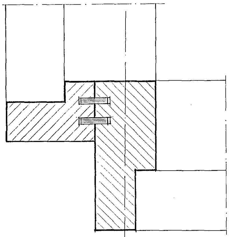
Snið A1-A1 M1:2
