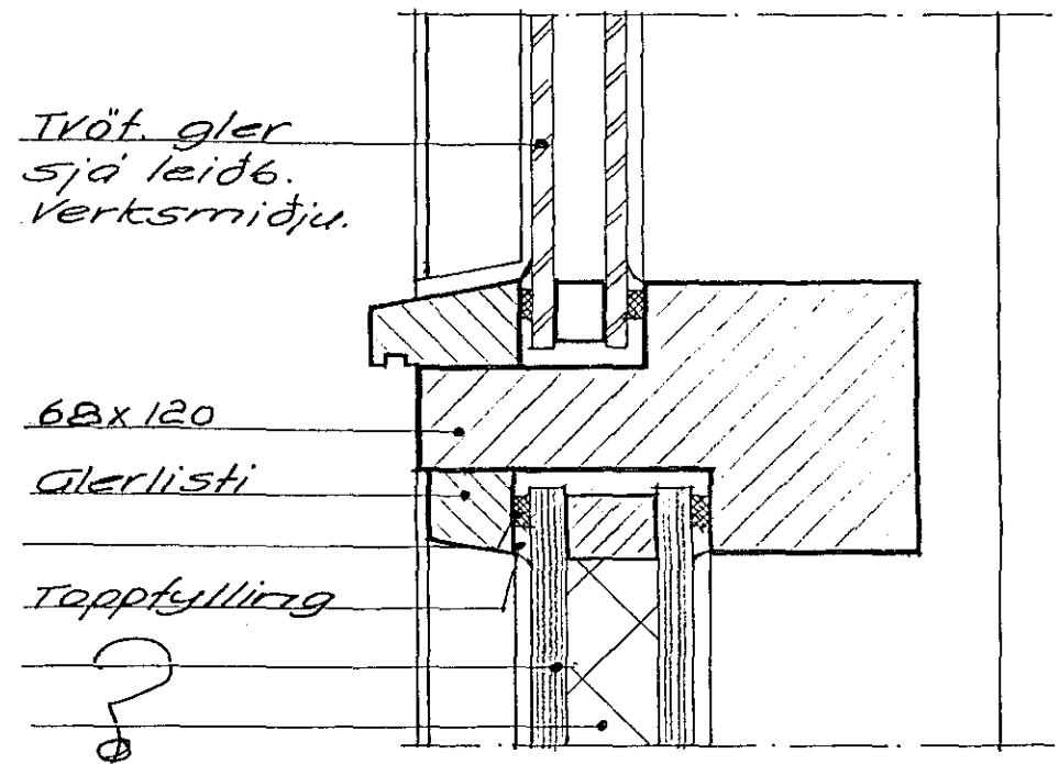
Snið A5-A5 M1:2
