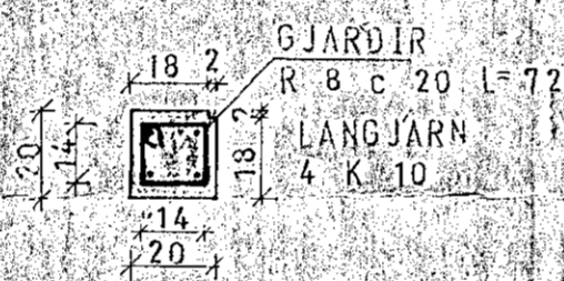
SÚLA S.13. 1:20
