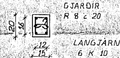
SÚLA S.15. 1:20
