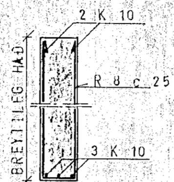
SNID A-A 1:20
