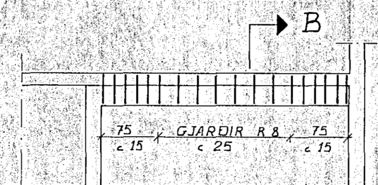
BITI B.1.3. 1:50
