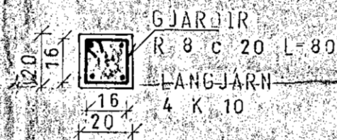
SÚLA S.14. 1:20
