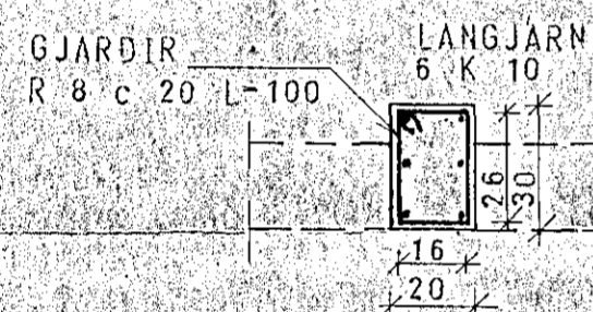
SÚLA S.11. 1:20
