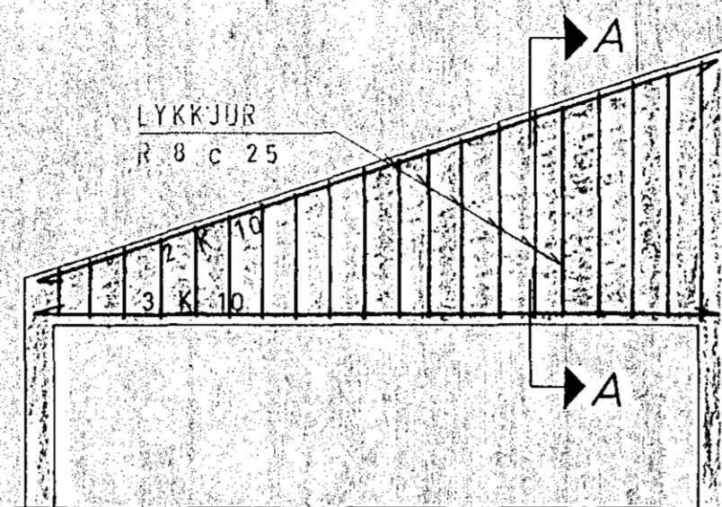
BITI B.12. 1:50
