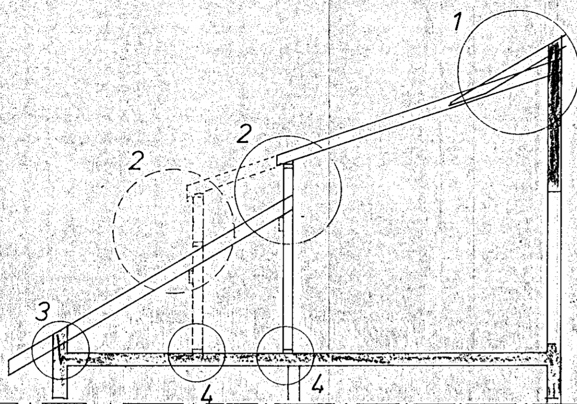
SNID B-B 1:50
