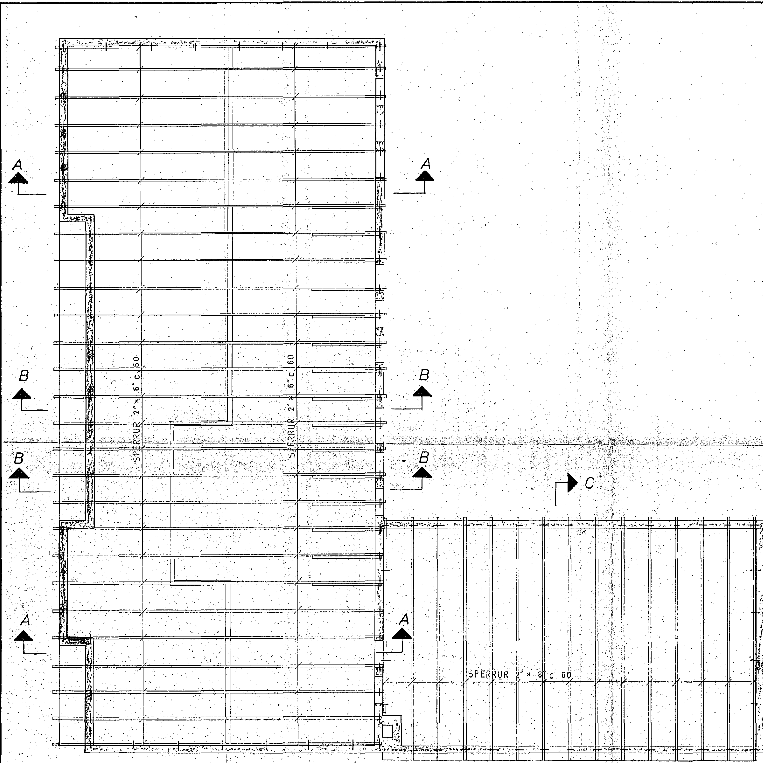
GRUNNMYND - RIS 1:50
