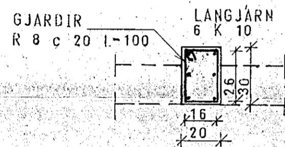
SÚLA S.11. 1:20
