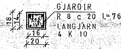
SÚLA S.12. 1:20
