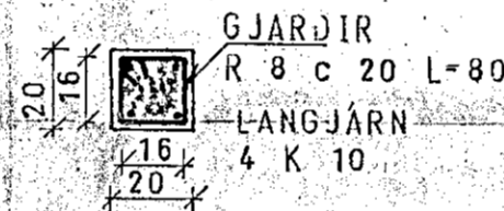
SÚLA S.14. 1:20
