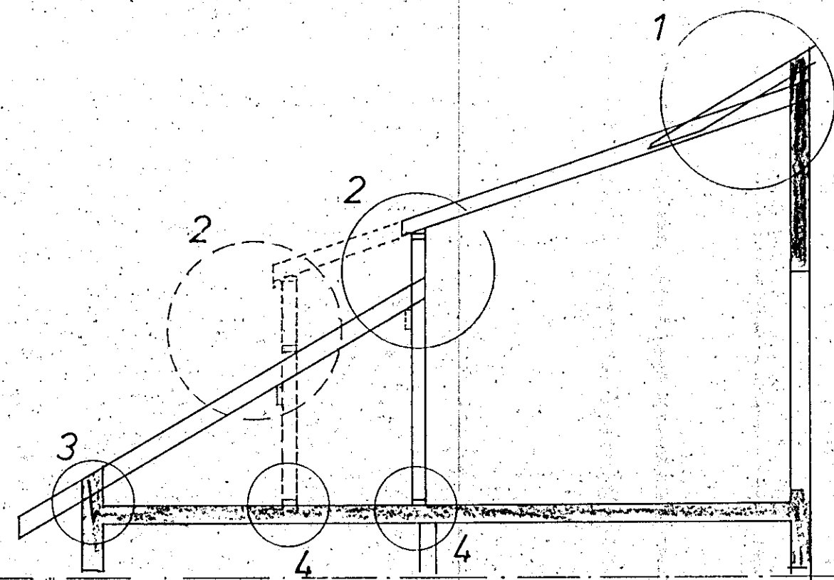
SNID B-B 1:50
