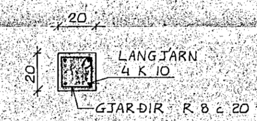
SÚLA S1 1:20
