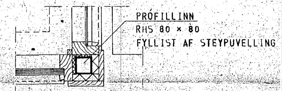
SERMYND 1 1:10
