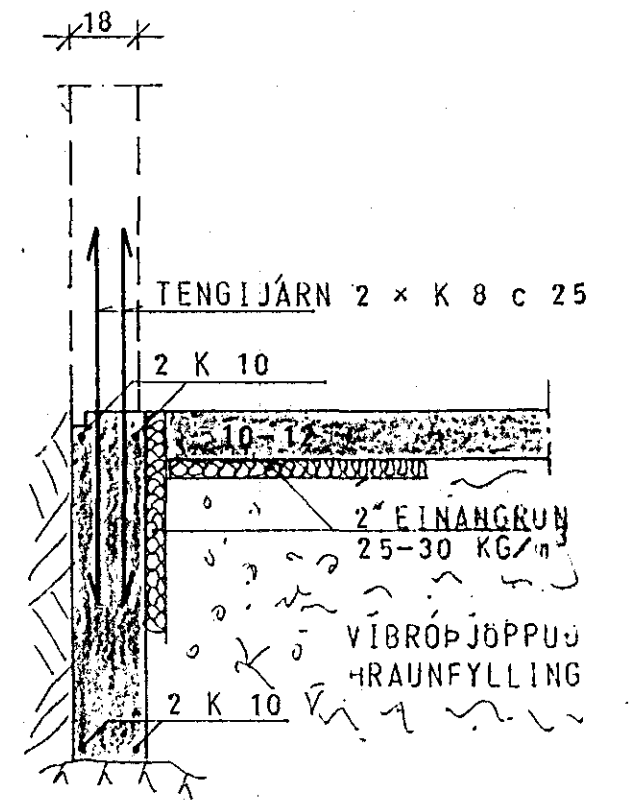
SNID Í ÚTVEGGI 1:20
