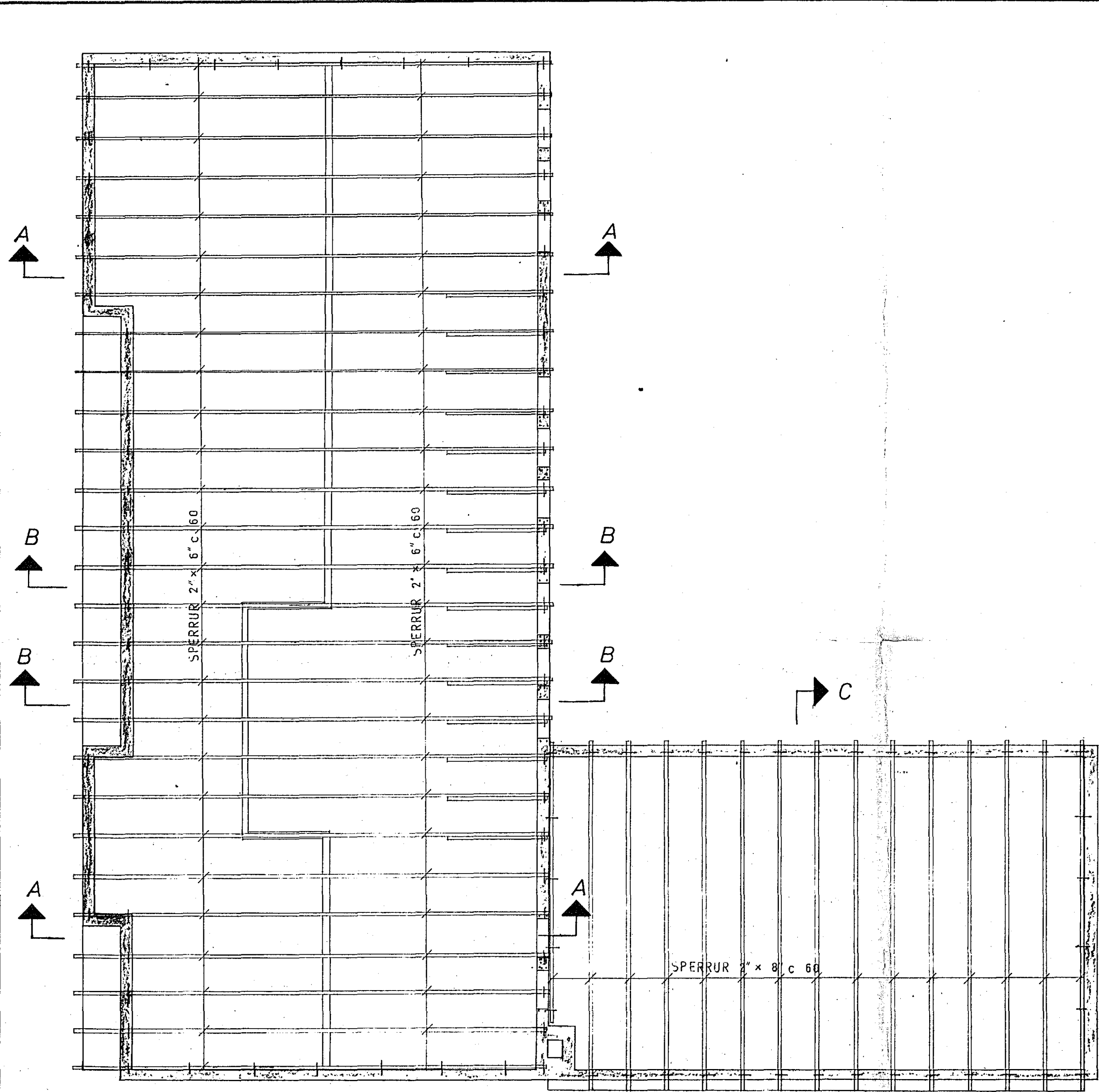
GRUNNMYND - RIS 1:50
