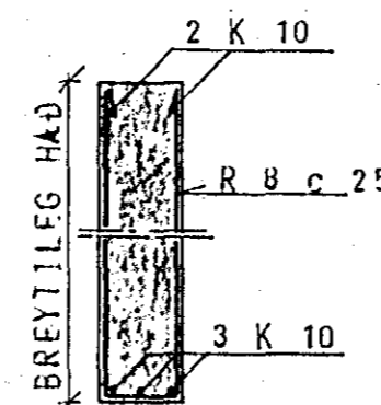
SNID A-A 1:20
