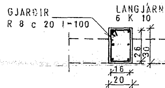
SÚLA S.1.1 1:20
