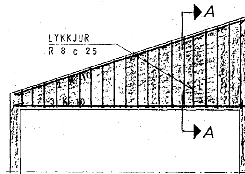
BITI B.1.2 1:50
