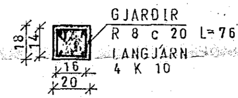
SÚLA S.1.2 1:20
