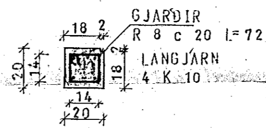
SÚLA S.1.3 1:20
