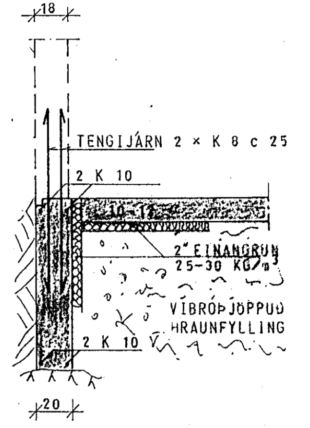
SNID Í ÚTVEGGI 1:20
